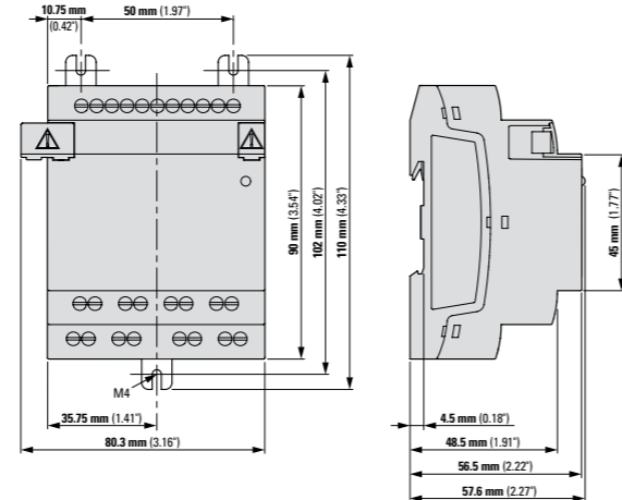
Большой модуль расширения
