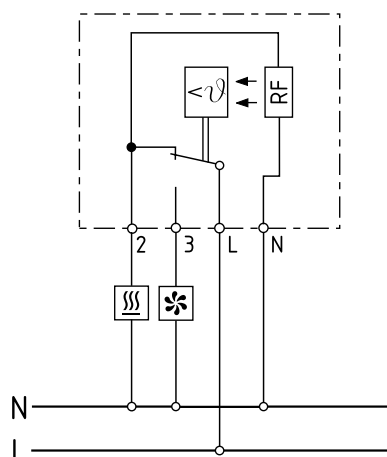
Схема подключения
