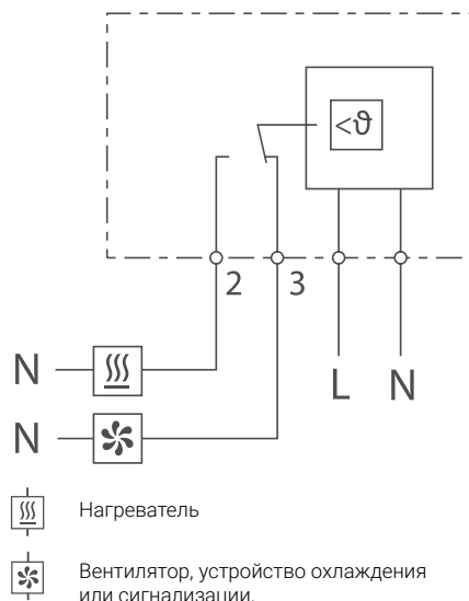
Схема подключения
