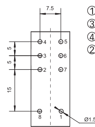
SRC08-P Вид снизу
