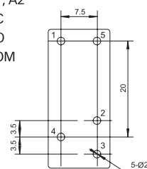
SRC05-P Вид снизу
