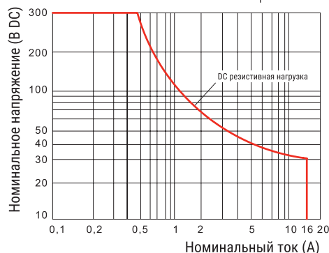
RKL1CO Макс. номинальная мощность
