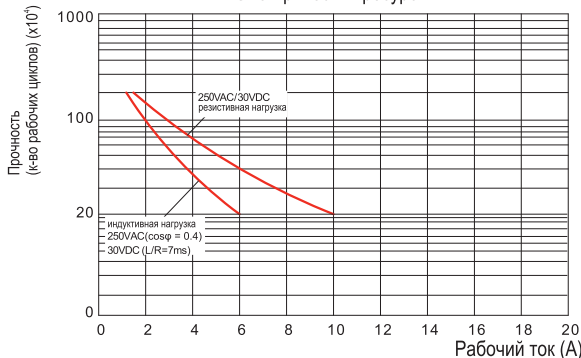
RKL2CO Электрический ресурс
