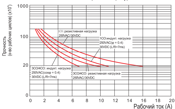
RKL1CO/3CO/4CO Электрический ресурс
