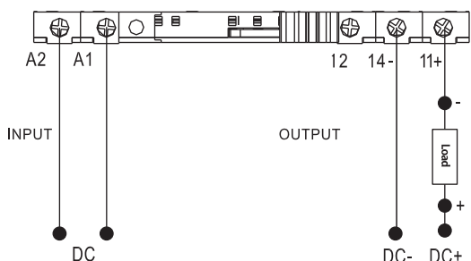
С колодкой SNB05-E-A Резистивная нагрузка
