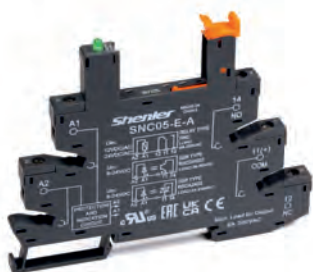
Цоколь
