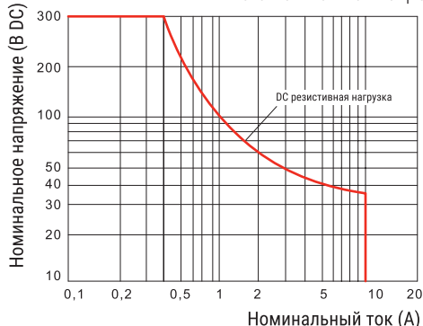
RKL2CO/3CO/4CO Макс. номинальная мощность
