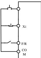
(d) Three-line running mode 1 (F00.03=3)
