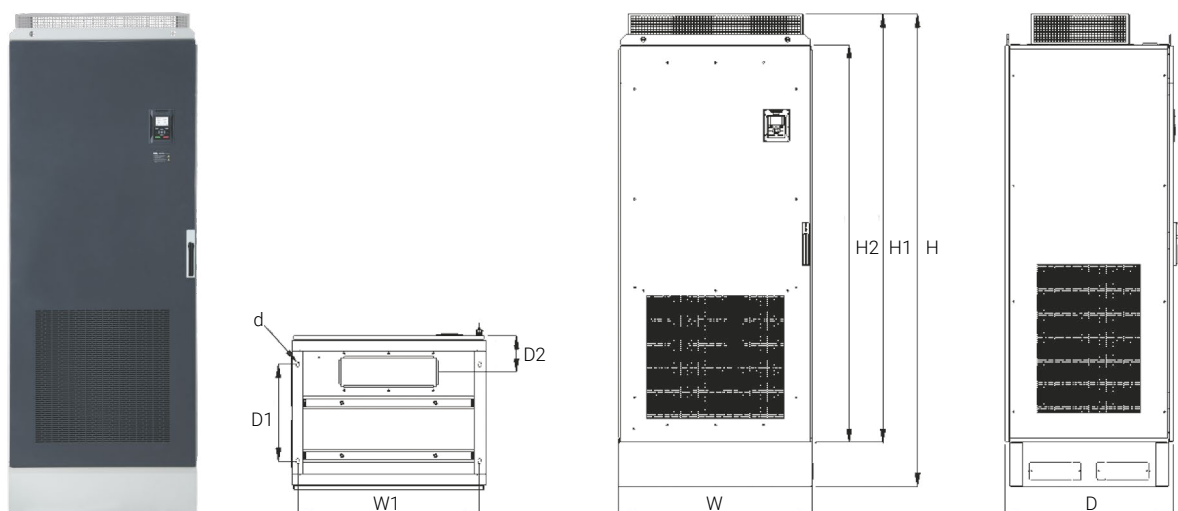
(С) Габаритные размеры моделей EM760C-450G/500P-3 – EM760C-560G/630P-3
