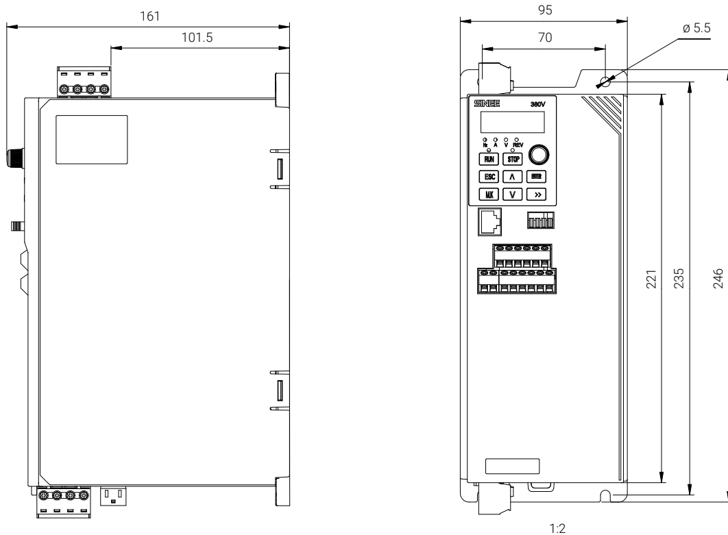
(B0) Размер E700-5R5-3B-EM700-7R5-3B
