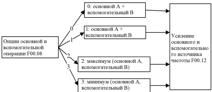
Рис. 1-4 Схематическая диаграмма настройки основных и вспомогательных операций
