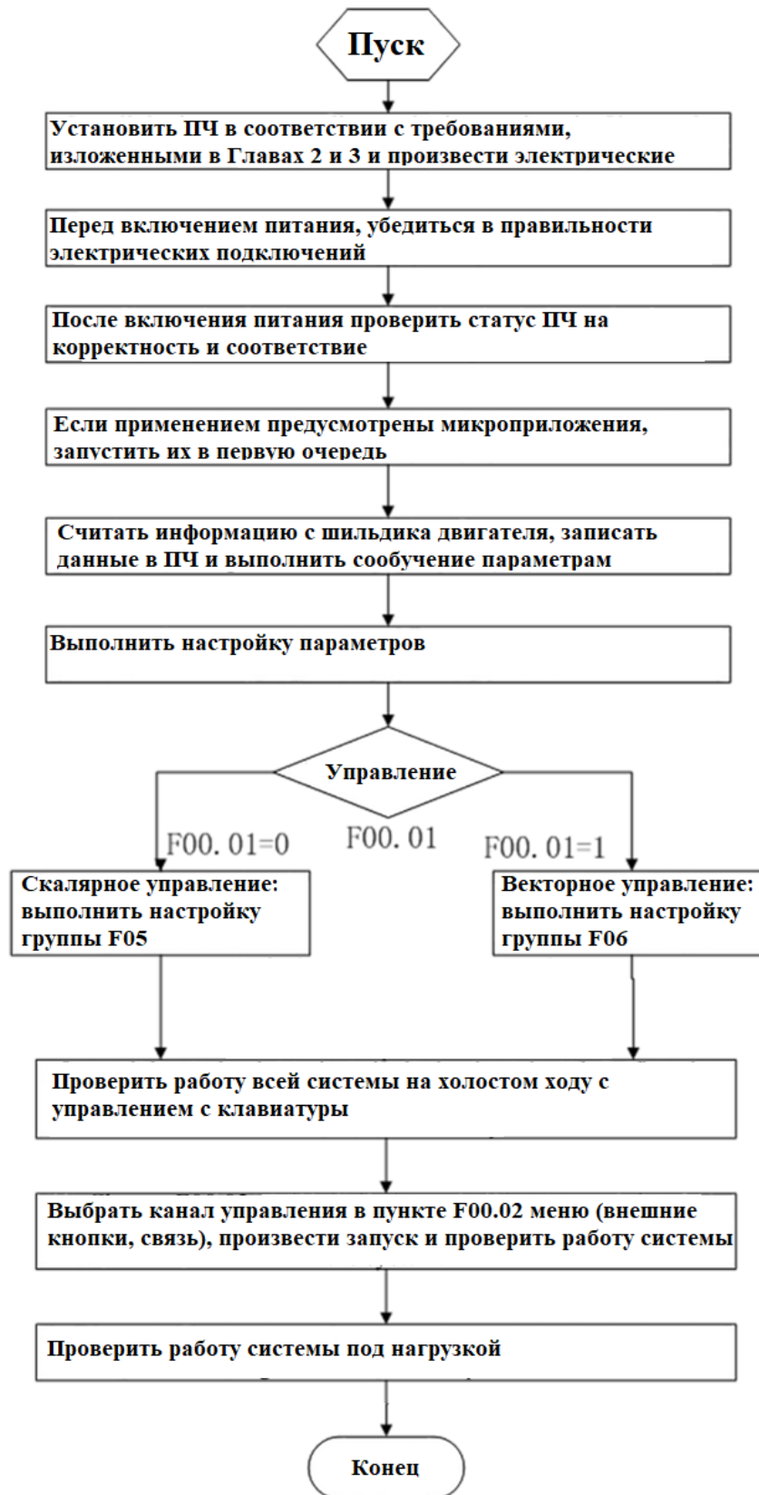
Рис. 5-1 Блок-схема процесса пуско-наладки ПЧ
