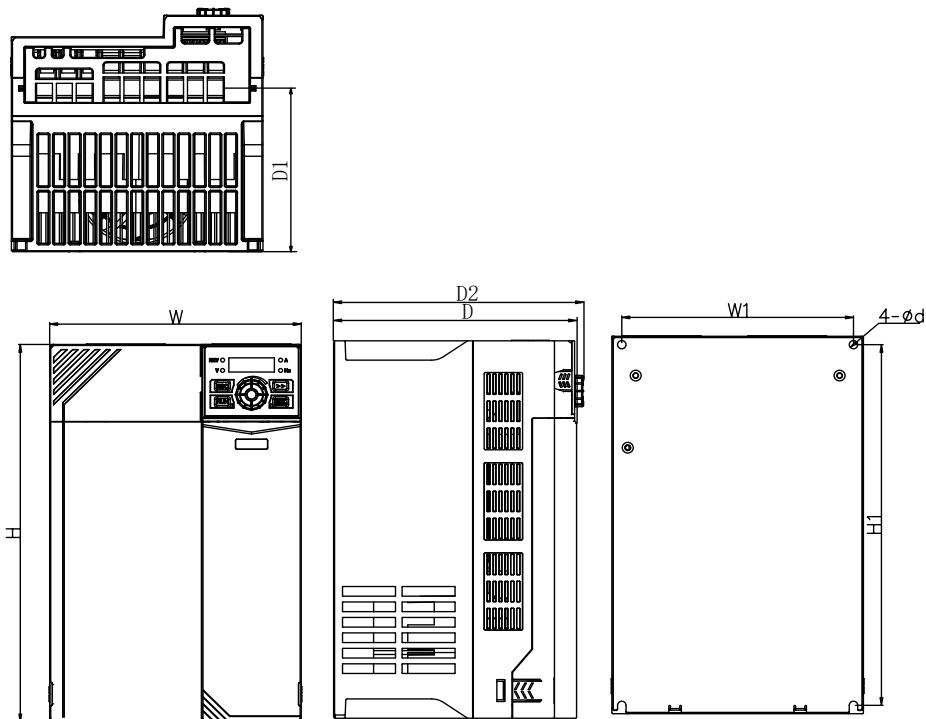
(a) Размеры моделей от EM730-0R7-3В до EM730-022-3В
