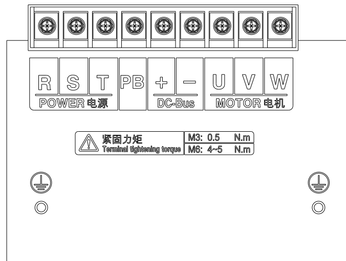
b) EM730-5R5-3B~EM730-022-3B
