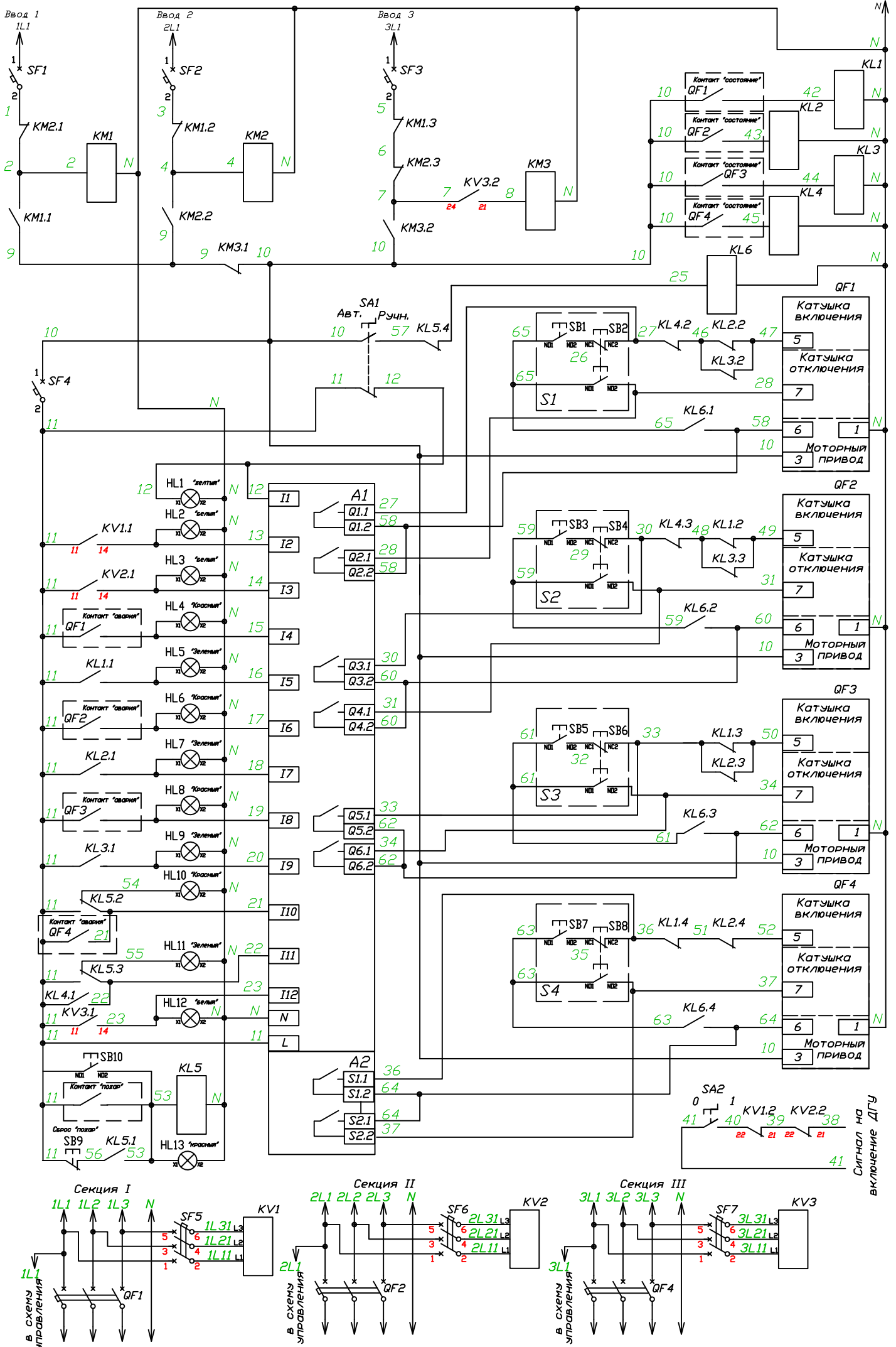
Схема подключения приводов силовых аппаратов приведена для моторных приводов DPX3 Legrand пауза между отключением-включением привода 3с
