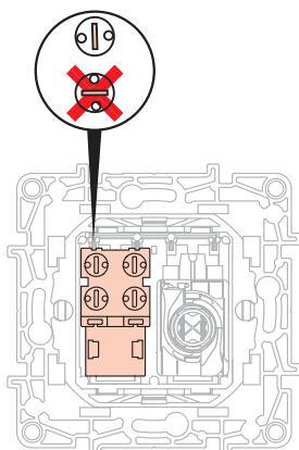
RJ 11 Подключение
