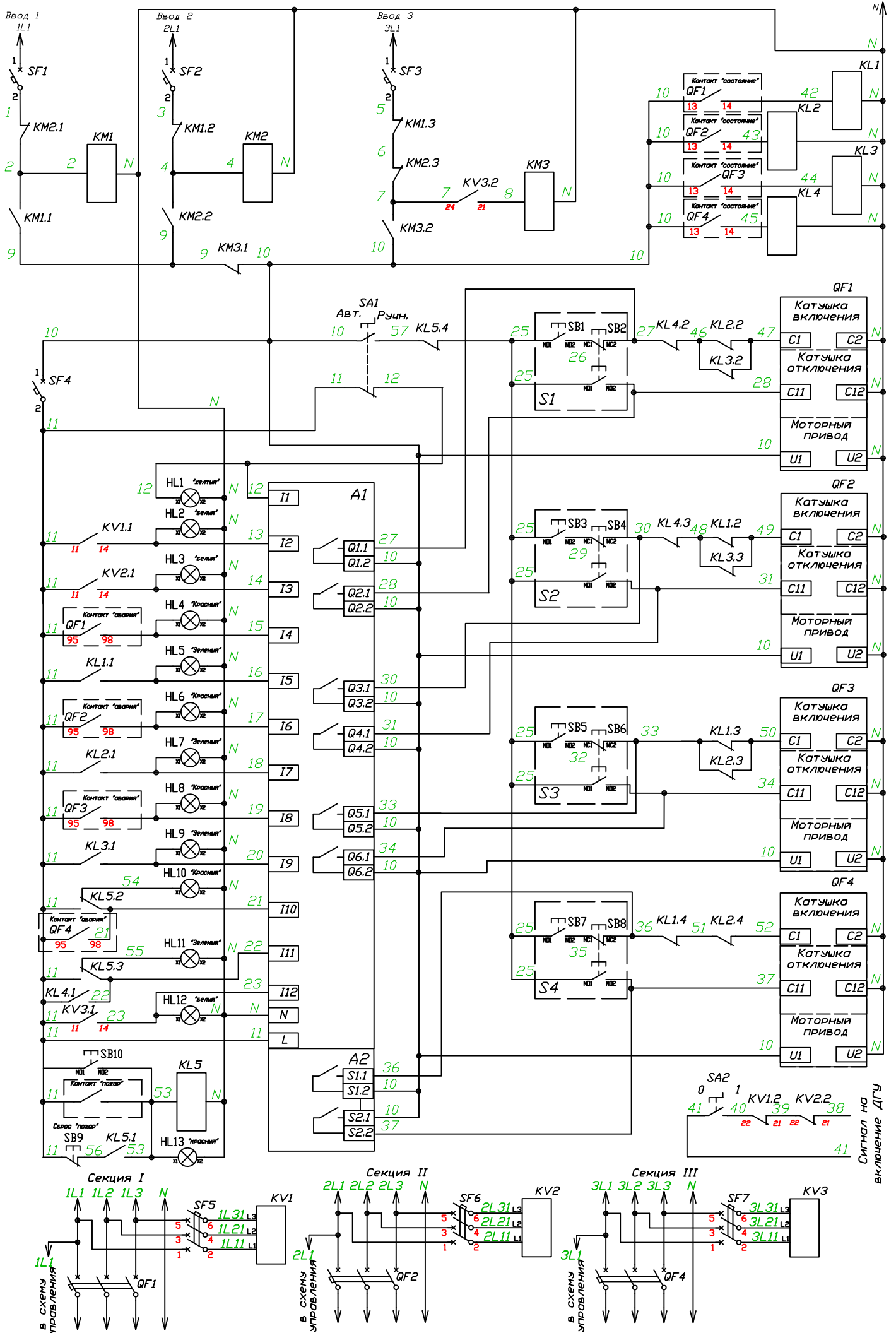
Схема подключения приводов силовых аппаратов приведена для моторных приводов АВВ для автоматов Еmax, X1, ТmaxТ7М и Еmax2, время завода пружины привода 3с. Маркировка клемм дополнительных контактов силовых автоматов проставлена для автоматов Еmax, для автоматов типа X1, Т7М и Еmax2 вместо 13-14 необходимо использовать 11-14, вместо 11-12 использовать 21-22.
