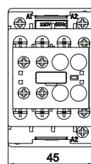
CNN 18+BP2(BP4)
