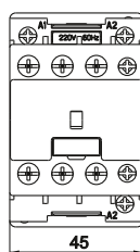
CNN 18
