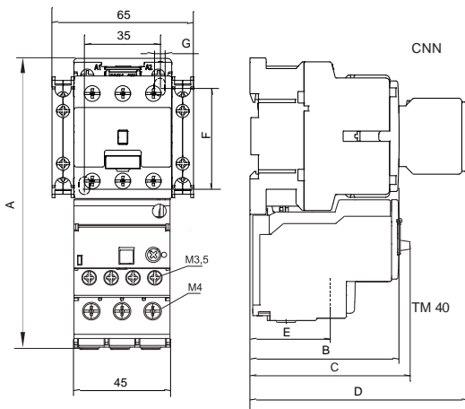
TM 40 + ASM 40
