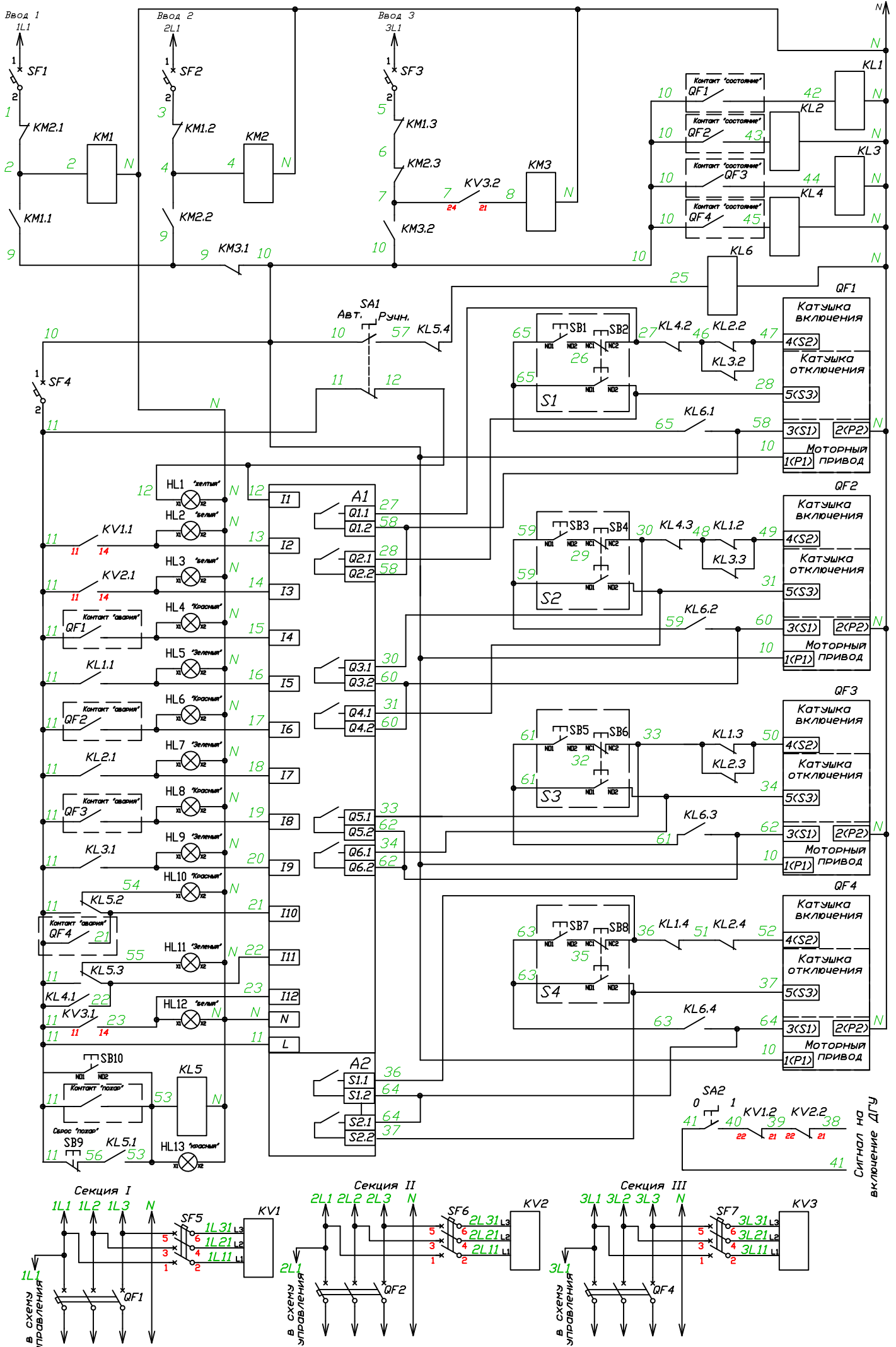
Схема подключения приводов силовых аппаратов приведена для моторных приводов Hyundai типа МДТ время паузы между отключением-включением привода 3с
