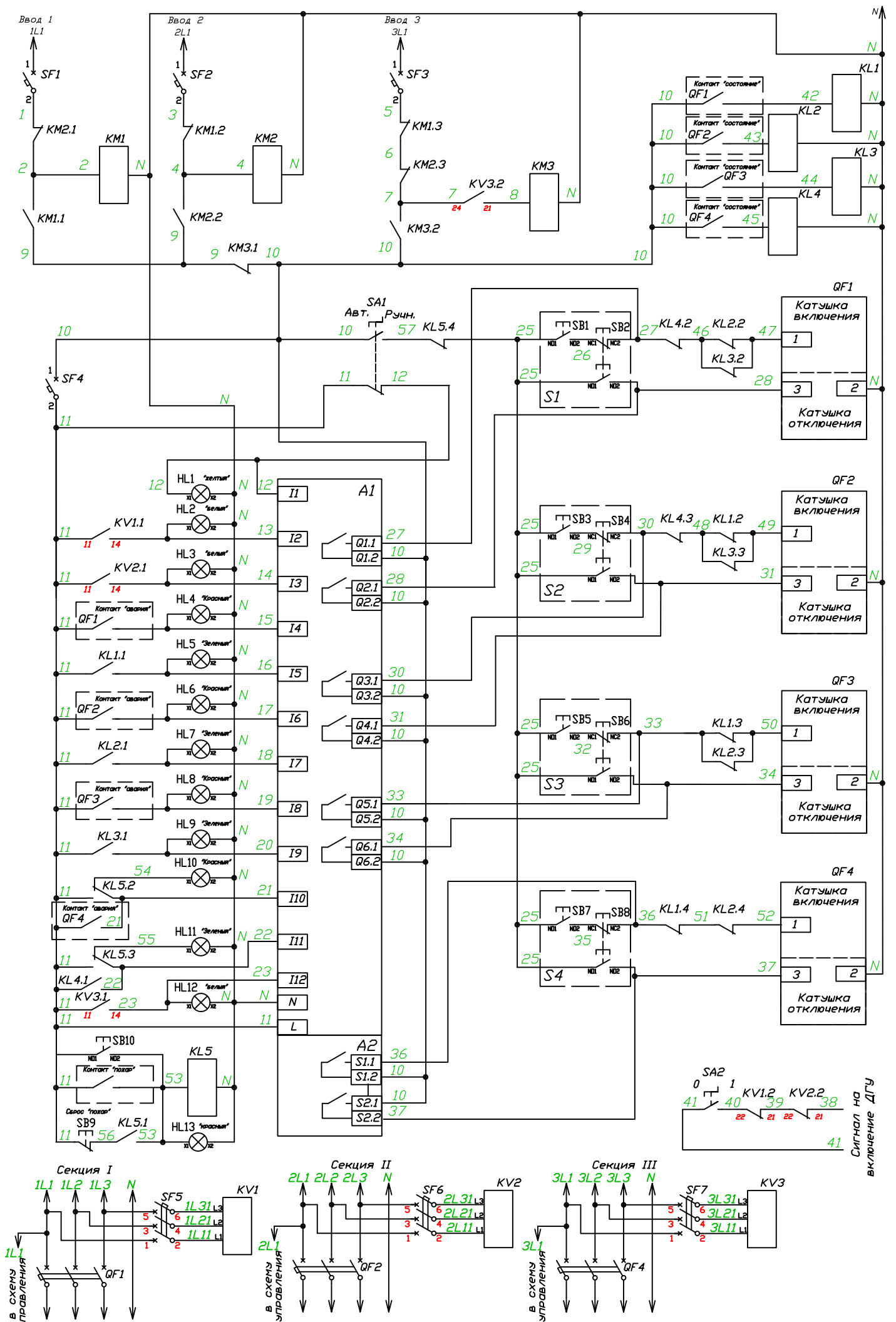
Схема подключения приводов силовых аппаратов приведена для моторных приводов Legrand DPX1250 (26123) длительность команды на включение должна быть не менее 4с; длительность команды на отключение должна быть не менее 6с.
