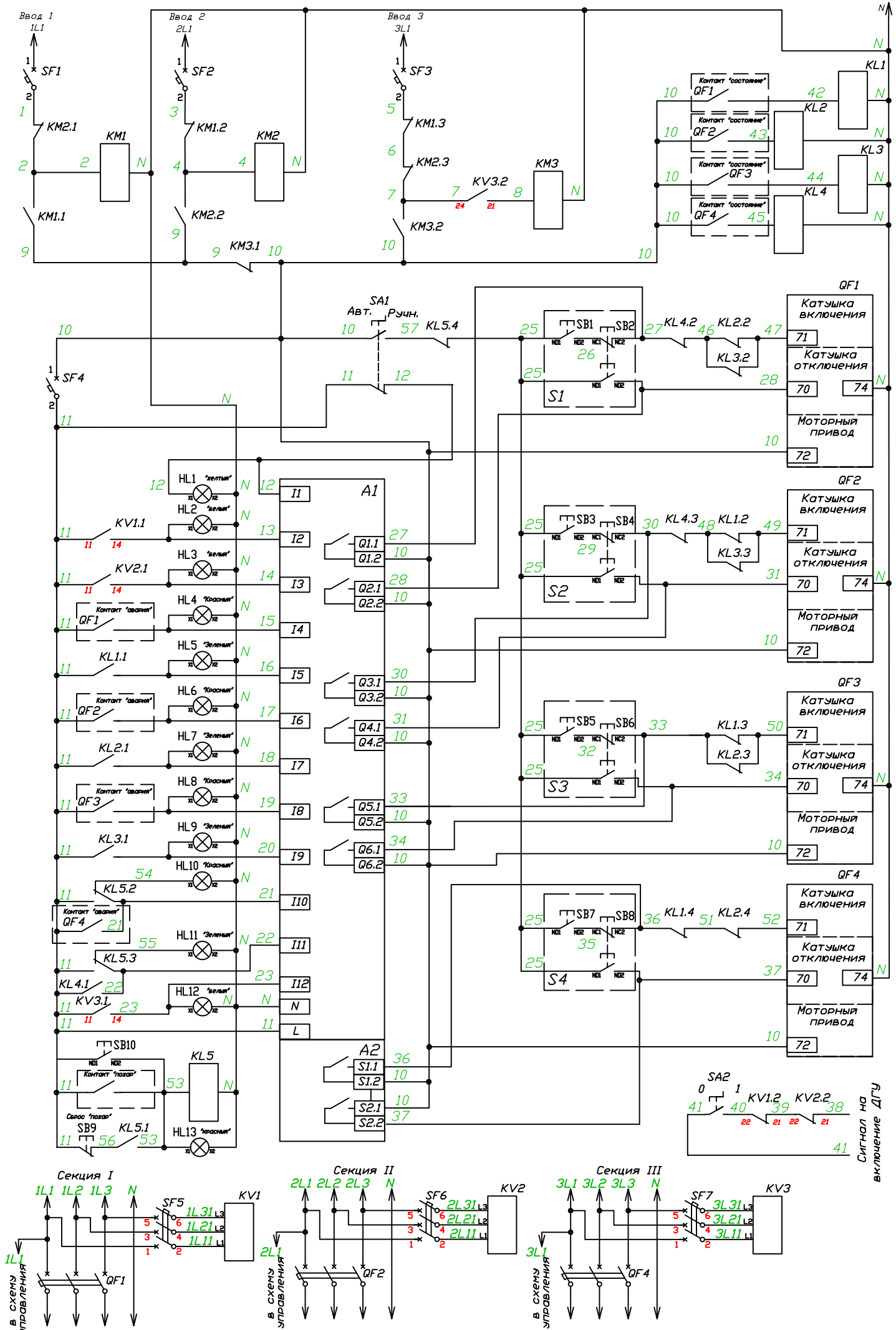
Схема подключения приводов силовых аппаратов приведена для моторных приводов MOELLER типов NZM2, NZM3, NZM4, время завода пружины привода 3с
