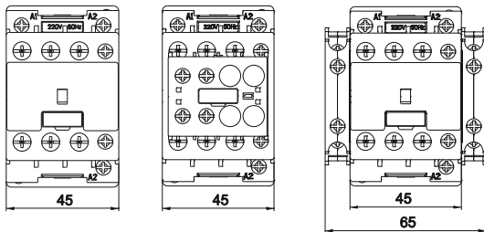
CNN 18+BP2(BP4)
