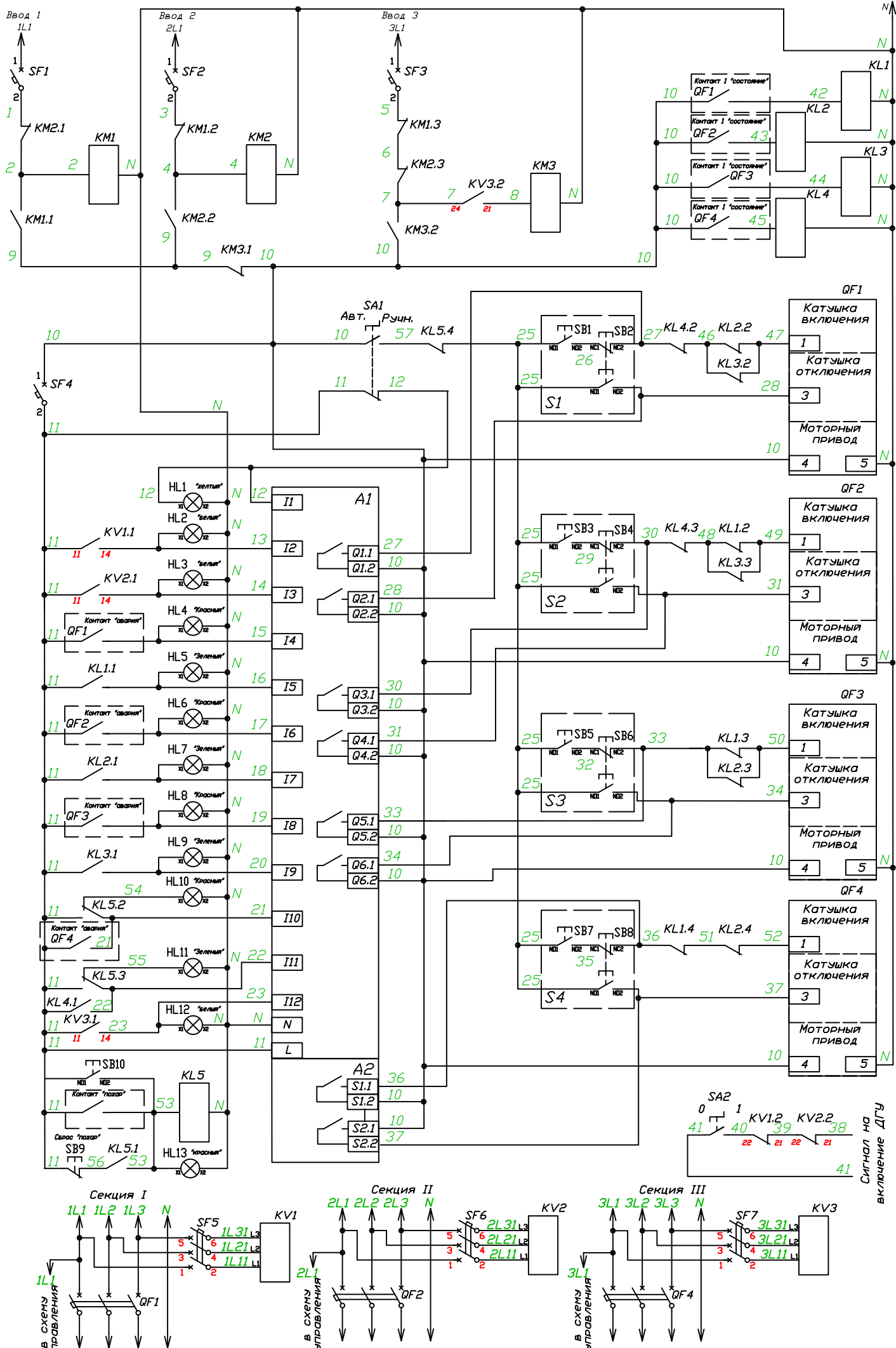
Схема подключения приводов силовых аппаратов приведена для моторных приводов ЭП40/43 для автоматических воздушных выключателей ВА88-40, ВА88-43. Время паузы между отключением и следующим включением 5с
