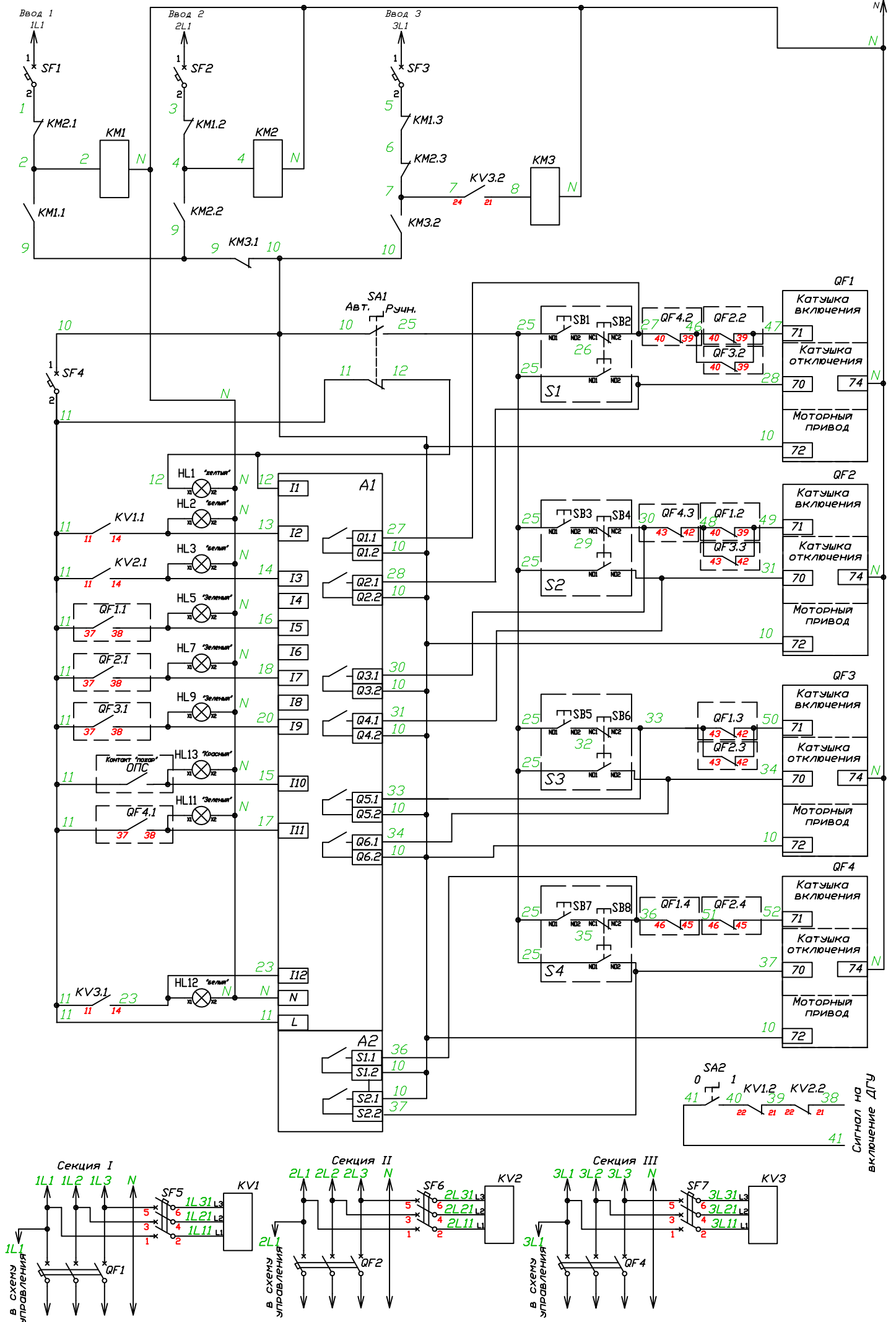
Схема подключения приводов силовых аппаратов приведена для моторных приводов ВА56, время завода пружины привода 3с
