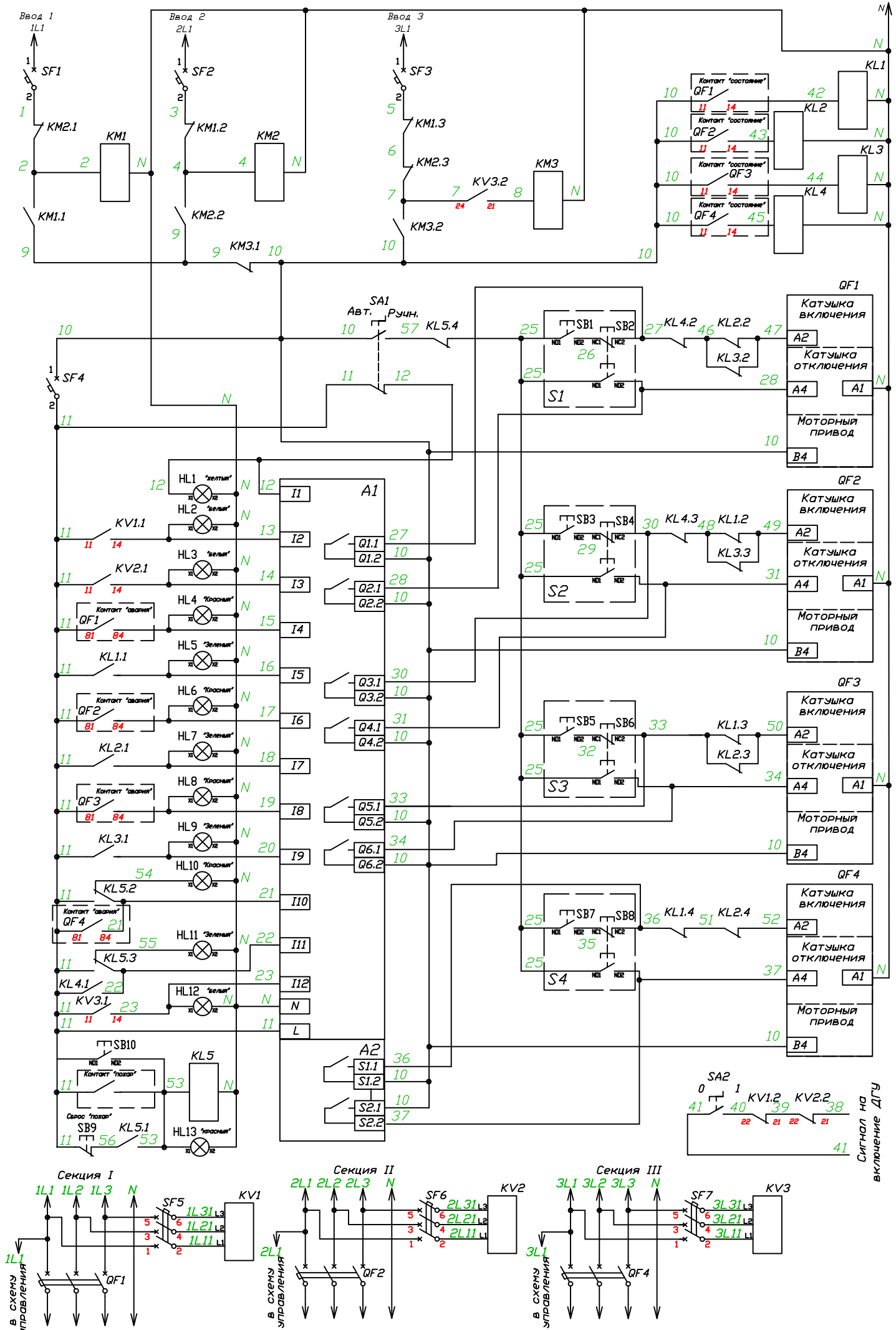
Схема подключения приводов силовых аппаратов приведена для моторных приводов SСHNEIDER ELECTRIC типов МТ100/160, МТ250, МТ400/630 время паузы отключения-включения 3с
