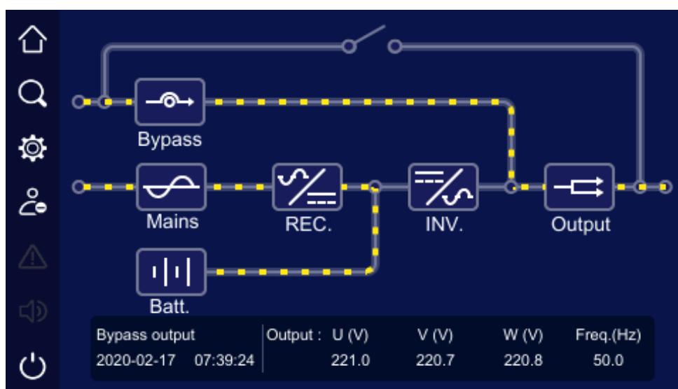
Рис 4.7 Питание нагрузки через байпас
