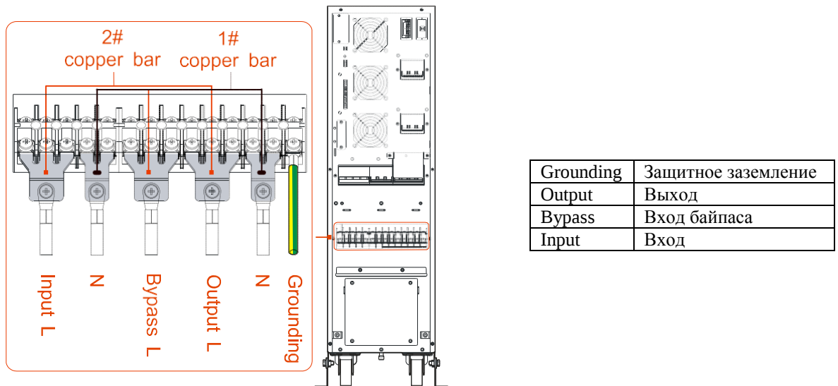
Рис. 3-16 Установка перемычек и подключение кабелей для 11 режима
