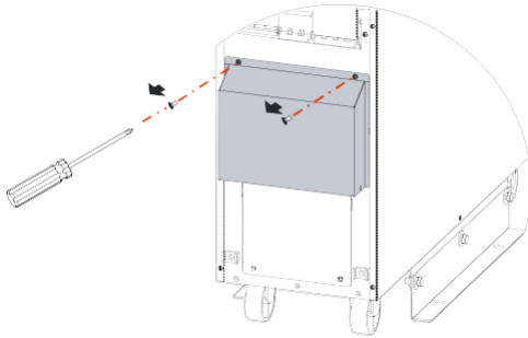
Рис. 3-12 Выверните винты крепления кабельной крышки
