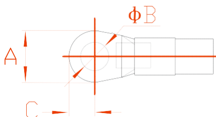
Рис3-1 Размеры кабельных наконечников
