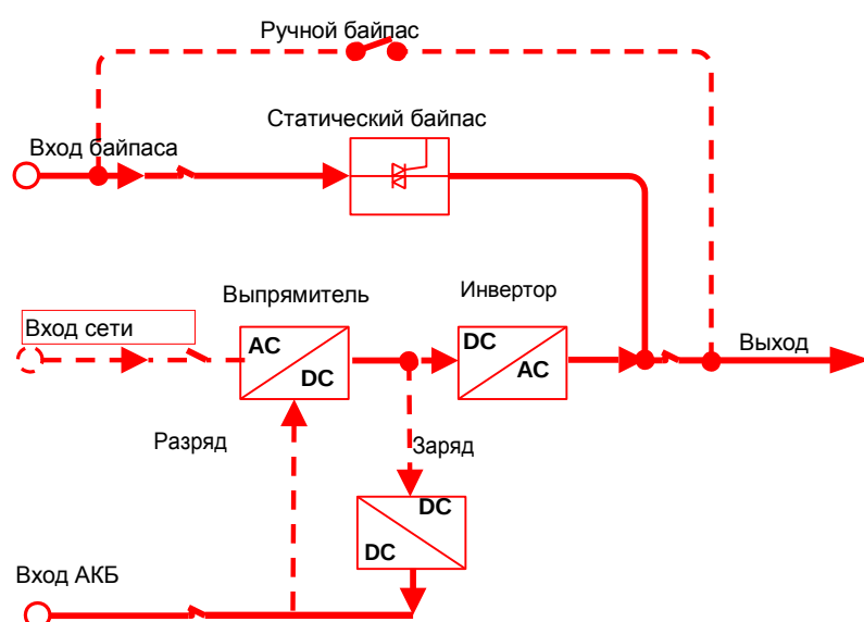
Рис 2-11 Режим работы через байпас ((жирная линия показывает поток энергии))
