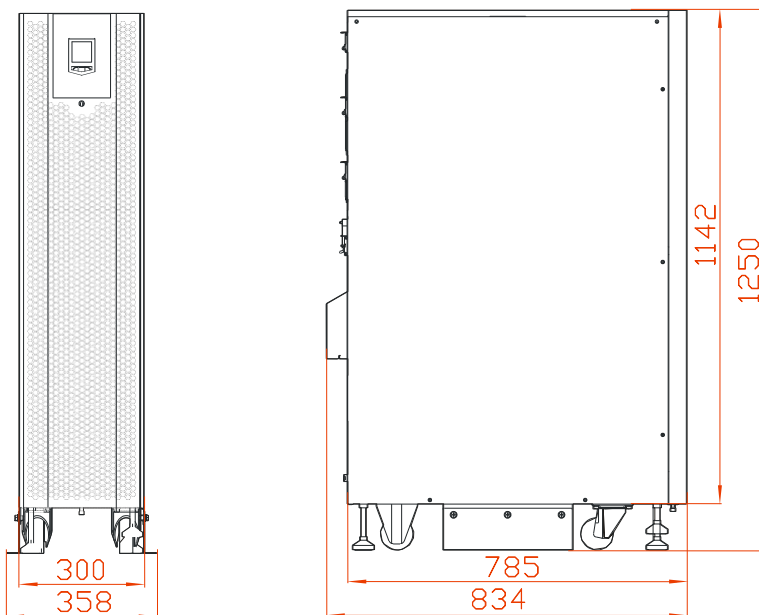
Рис. 3-7 Внешние размеры ИБП 30/30S/40/40S
