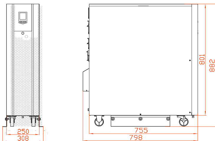
Рис. 3-6 Внешние размеры ИБП 10/10S/15/15S/20/20S
