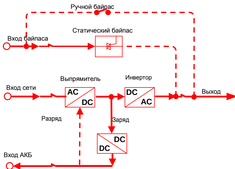
Рис 2-9 Нормальный режим работы от сети (жирная линия показывает поток энергии)
