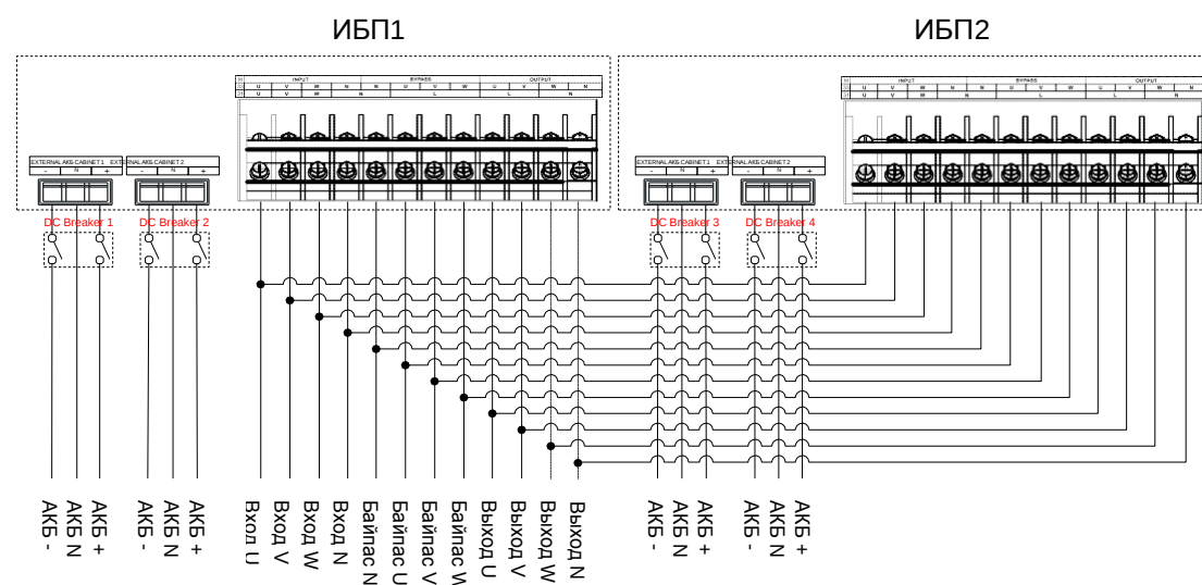
Рис. 3-29 30/30S/40/40S диаграмма подключения для 33 режима параллельной системы
