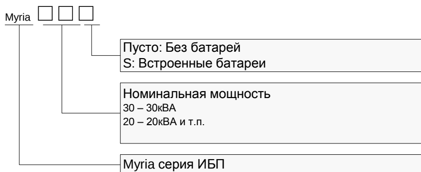
Рис2-1 Условное обозначение
