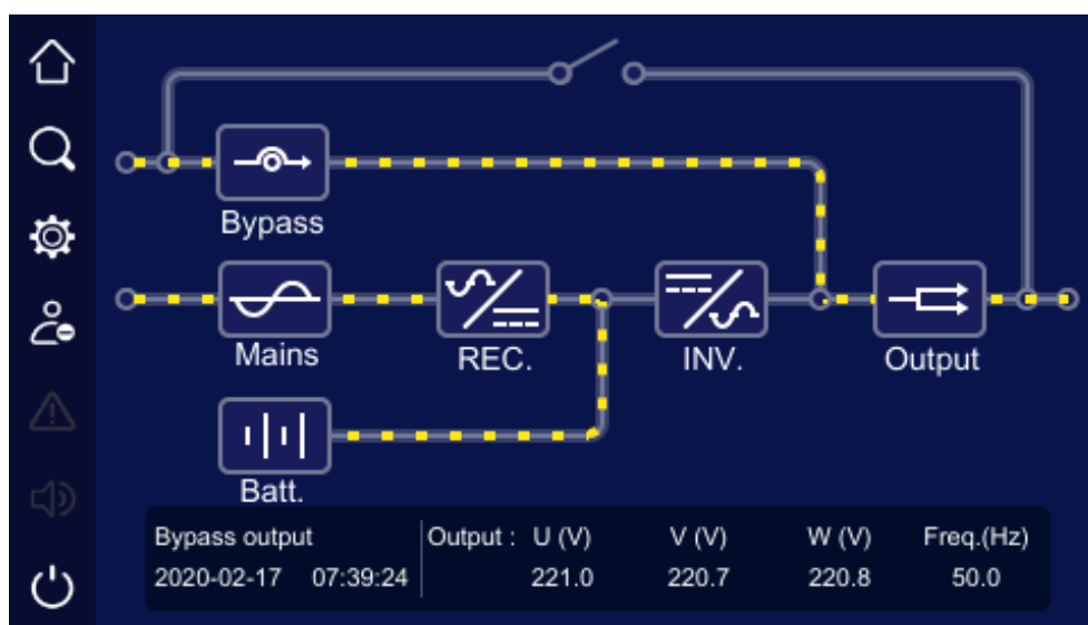
Рис 4.4 Без передачи энергии
