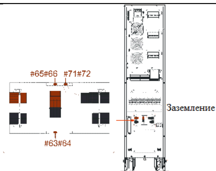
Рис. 3-20 Подключение установочной перемычки по умолчанию
