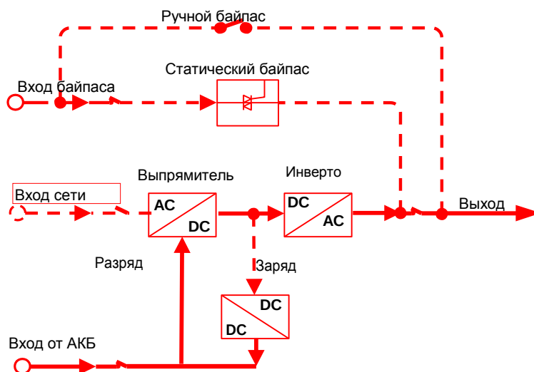
Рис 2-10 Режим работы от АКБ (жирная линия показывает поток энергии)
