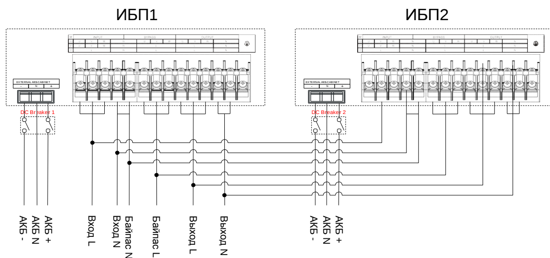
Рис. 3-28 10/10S/15/15S/20/20S диаграмма подключения для 11 режима параллельной системы
