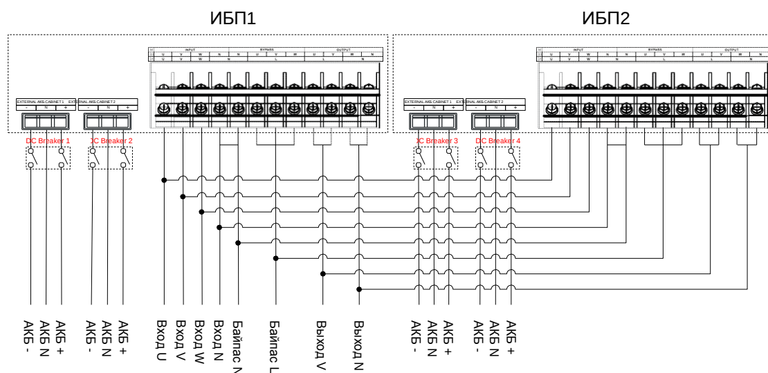
Рис. 3-30 30/30S/40/40S диаграмма подключения для 31 режима параллельной системы
