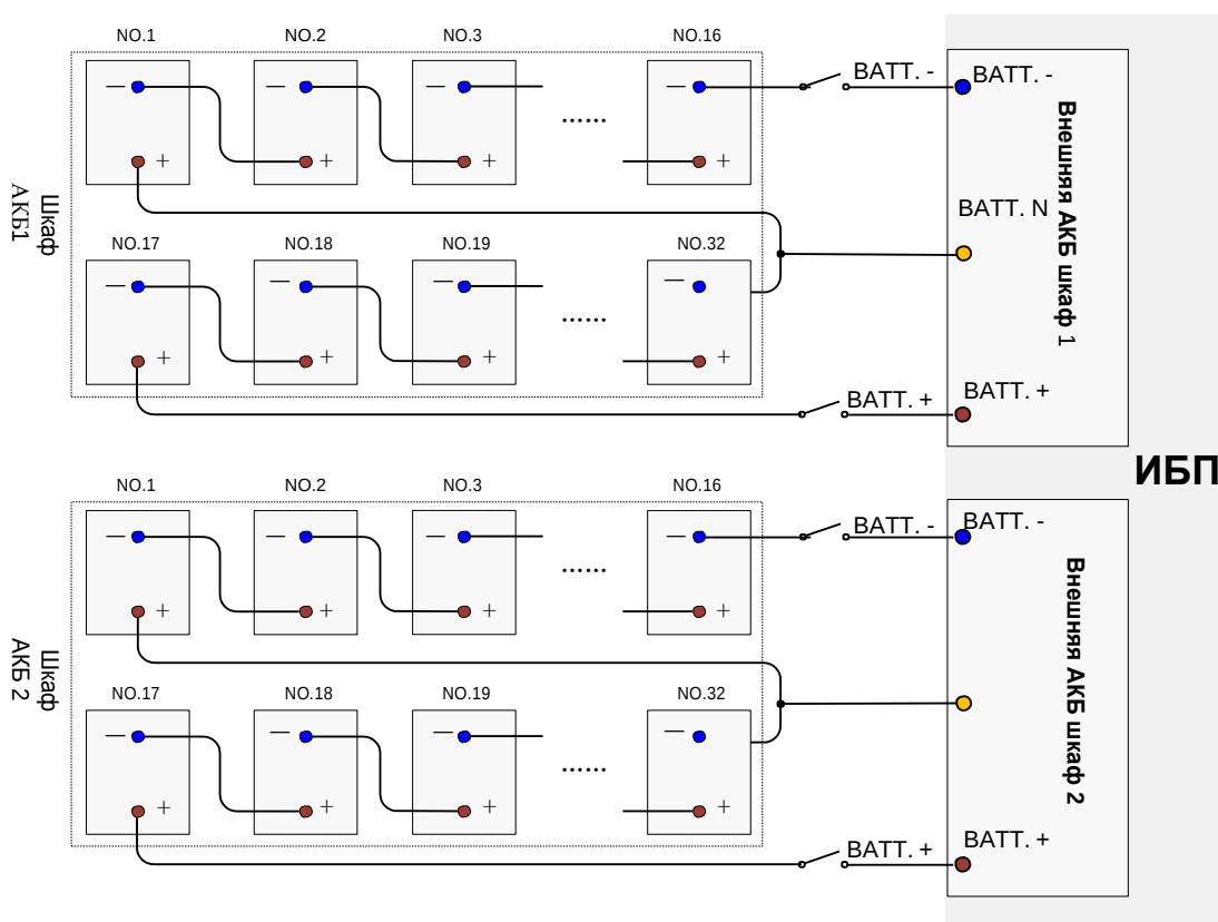
Рис. 3-25 Диаграмма подключения двух батарейных шкафов
