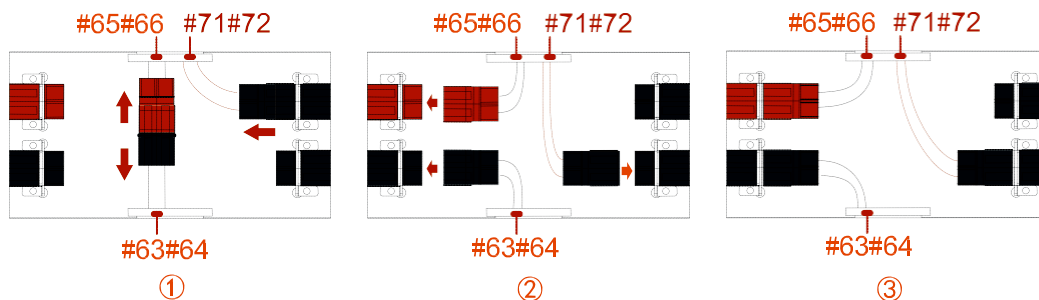
Рис. 3-22 Подключение установочной перемычки для 31 режима
