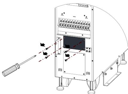
Рис. 3-18 Открутите винты, крепящие крышку отсека установочной перемычки
