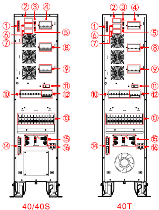
Рис 2-7 Вид задней панели моделей 40/40S
