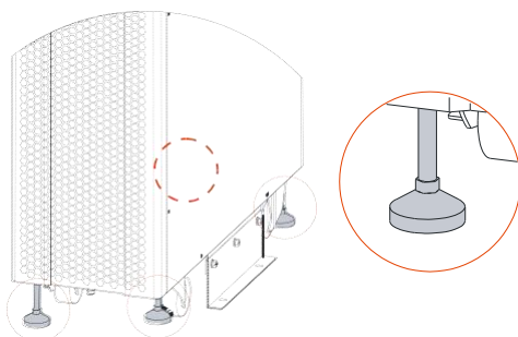
Рис. 3-11 Вкрутите поддерживающие опоры шкафа ИБП 30/30S/40/40S
