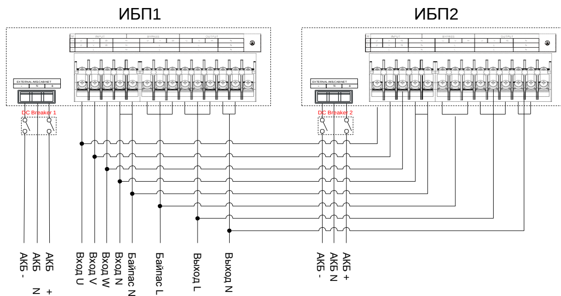
Рис. 3-27 10/10S/15/15S/20/20S диаграмма подключения для 31 режима параллельной системы
