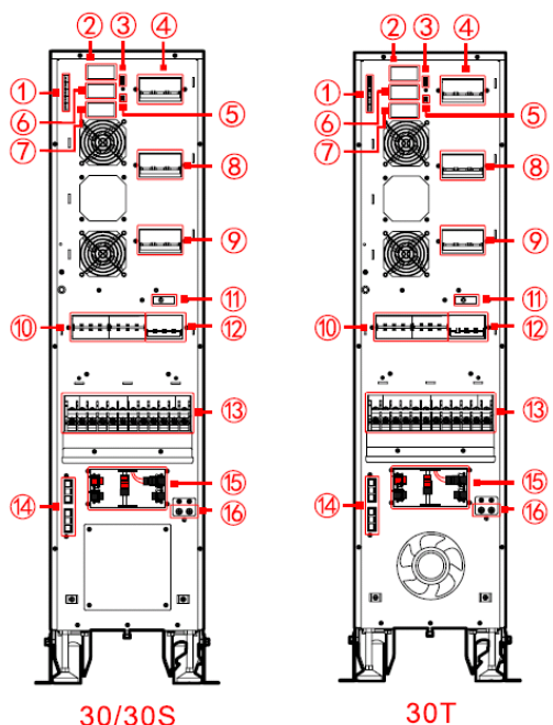
Рис 2-6 Вид задней панели моделей 30/30S
