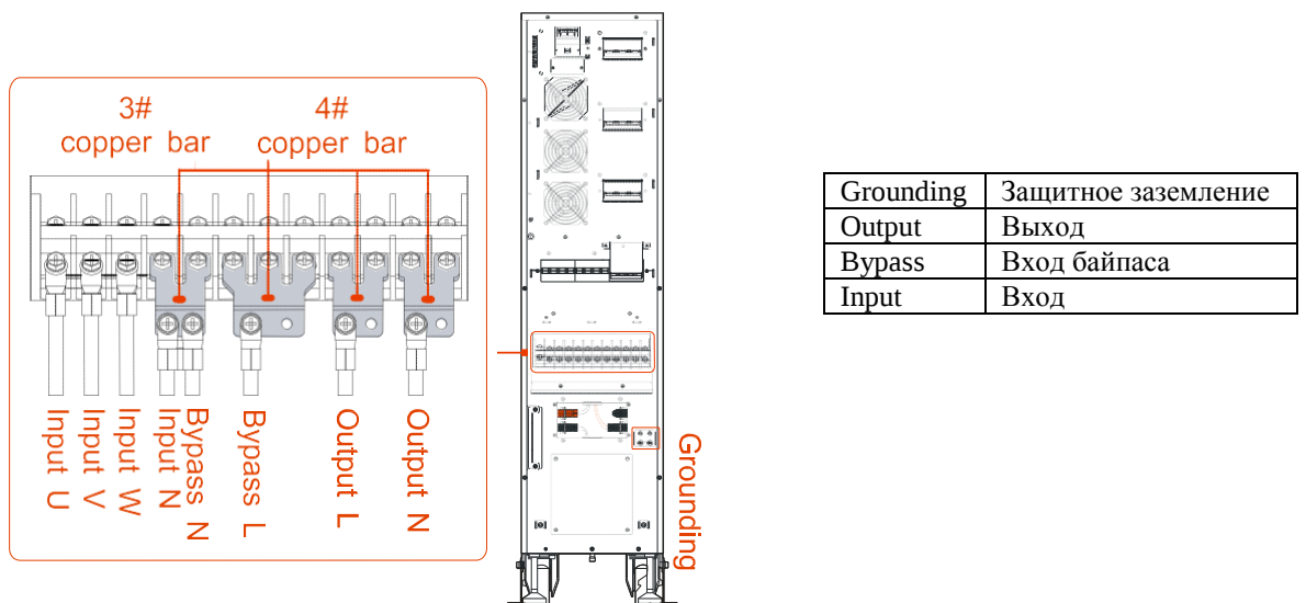
Рис. 3-23 Медные перемычки и диаграмма подключения для 31 режима
