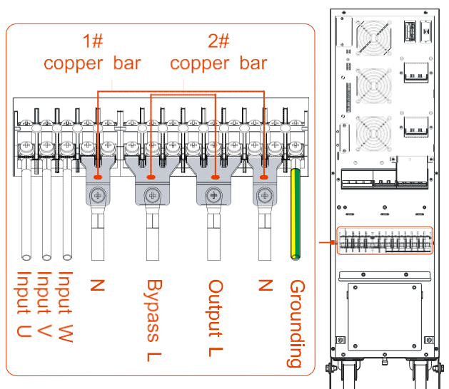
Рис. 3-15 Установка перемычек и подключение кабелей для 31 режима
