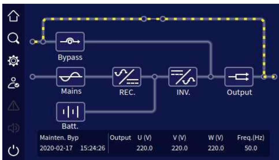
Рис 4.9 Работа через сервисный байпас
