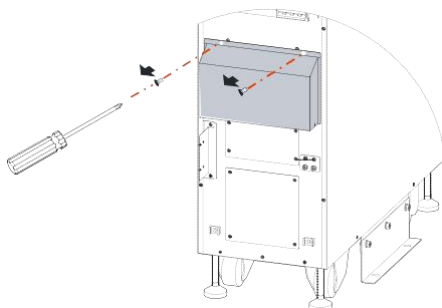
Рис. 3-17 Открутите винты кабельной крышки
