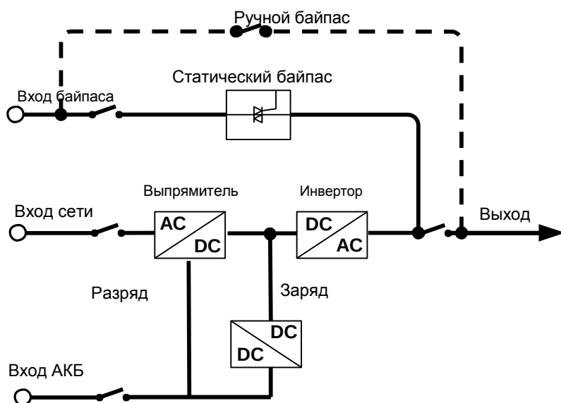
Рис. 2-8 Функциональная диаграмма
