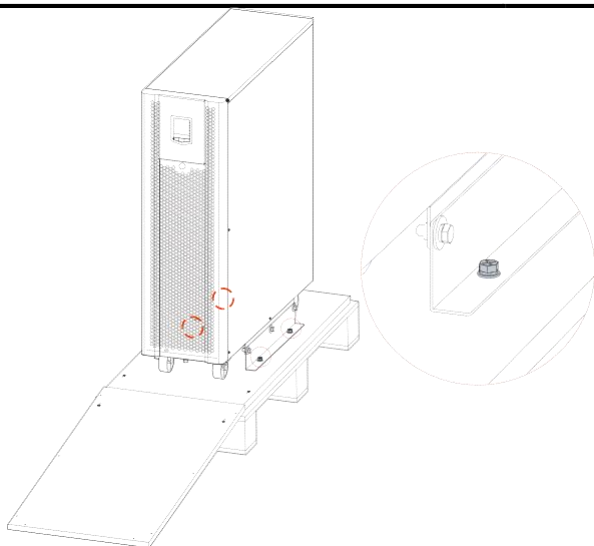
Рис. 3-4 Расположение крепёжных болтов
