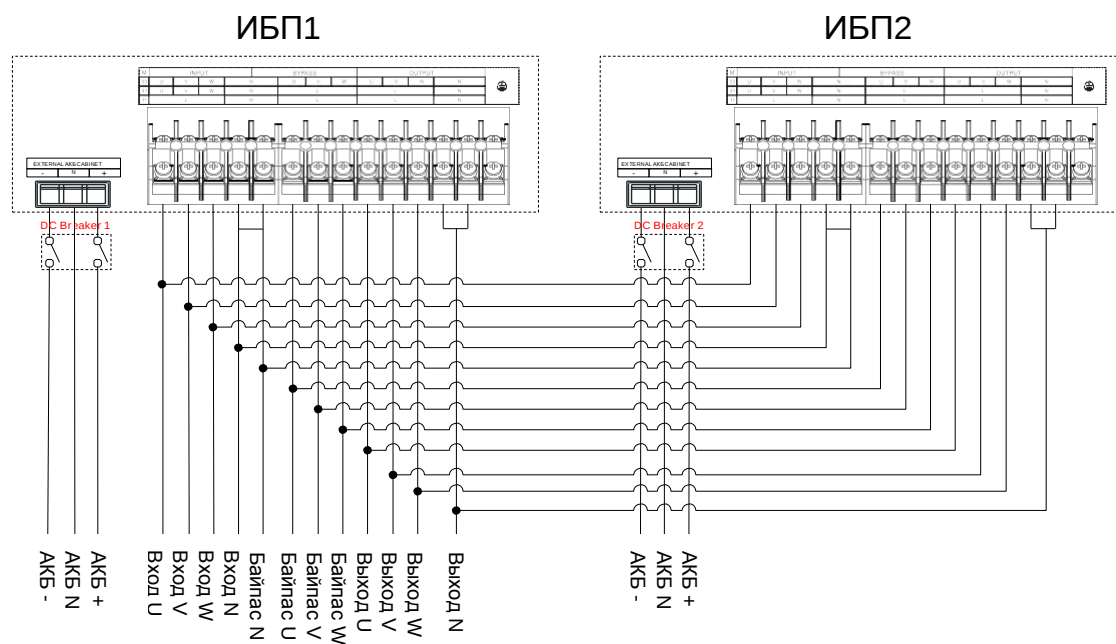
Рис. 3-26 10/10S/15/15S/20/20S диаграмма подключения 33 режим для параллельной системы
