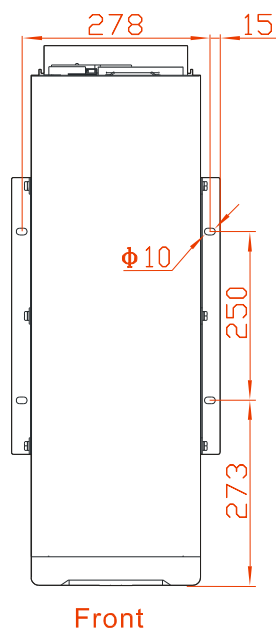
Рис. 3-8 10/10S/15/15S/20/20S отверстия для монтажа в раме ИБП (вид сверху)
