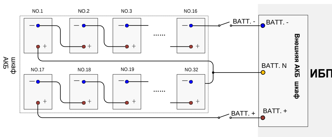
Рис. 3-24 Диаграмма подключения одного батарейного шкафа
