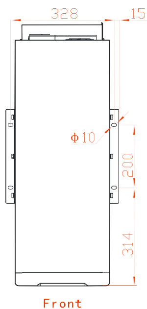
Рис. 3-9 30/30S/40/40S отверстия для монтажа в раме ИБП (вид сверху)
