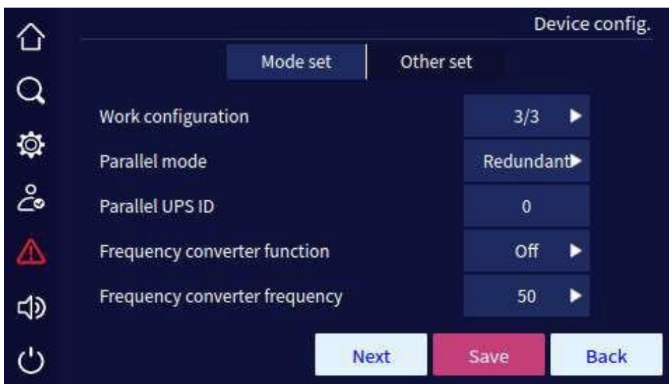
Рис 4.45 Страница настроек 1
