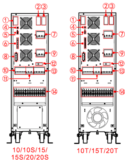
Рис 2-5 Вид задней панели моделей 10/10S/15/15S/20/20S
