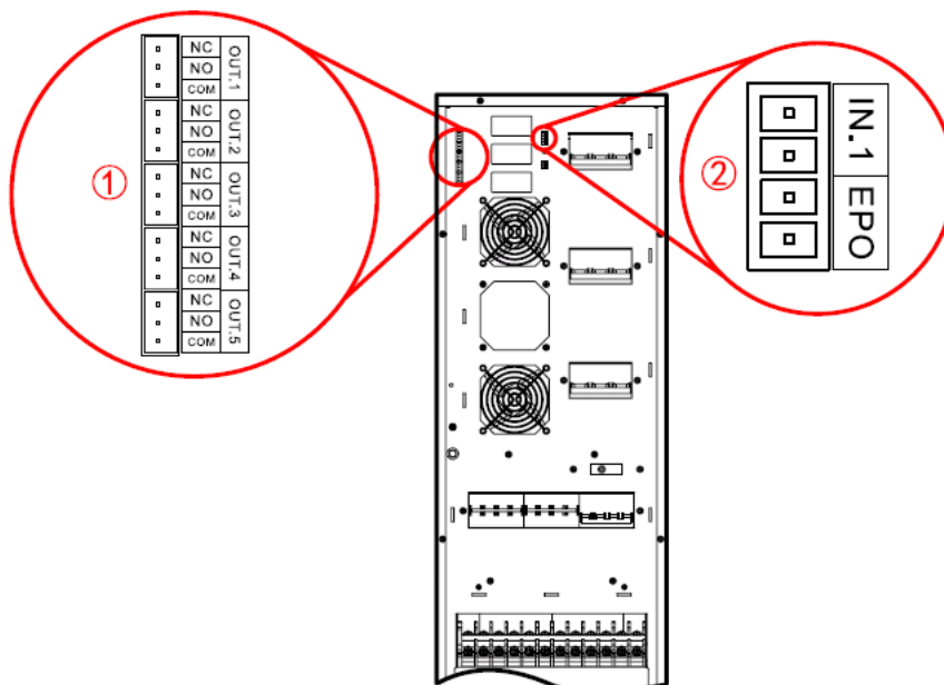
Рис 2-14 Расположение сухих контактов для ИБП 30/30S/40/40S
