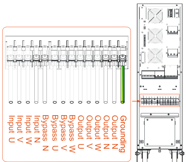
Рис. 3-14 Диаграмма подключения для 33 режима
