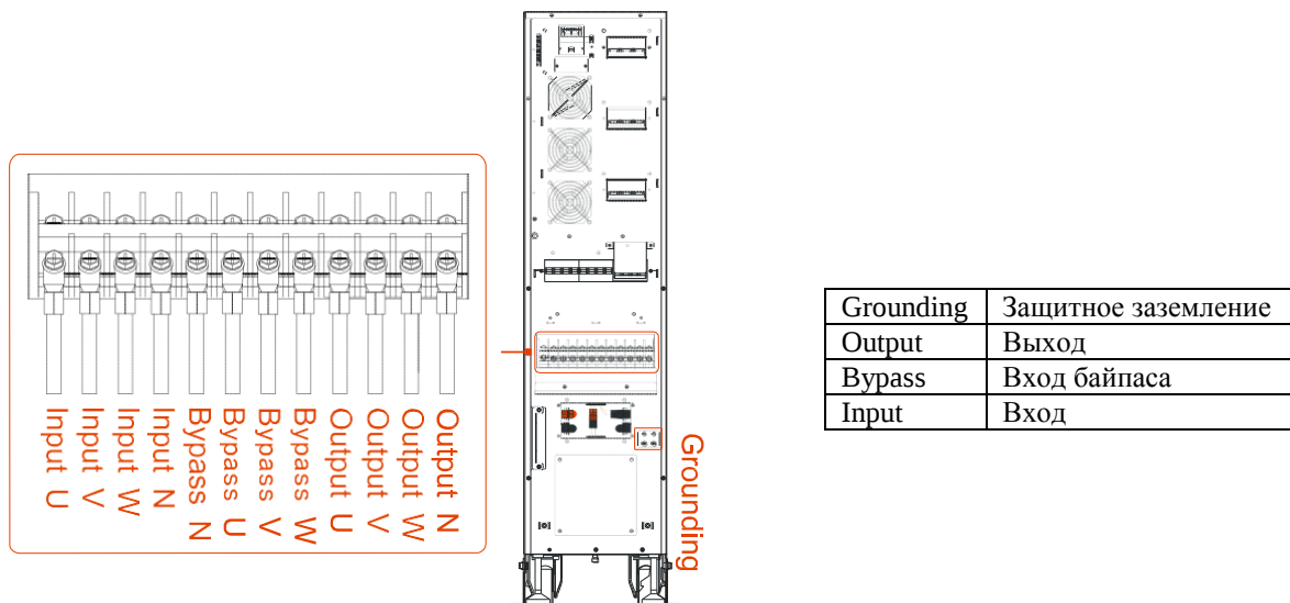
Рис. 3-21 Диаграмма подключения для 33 режима
