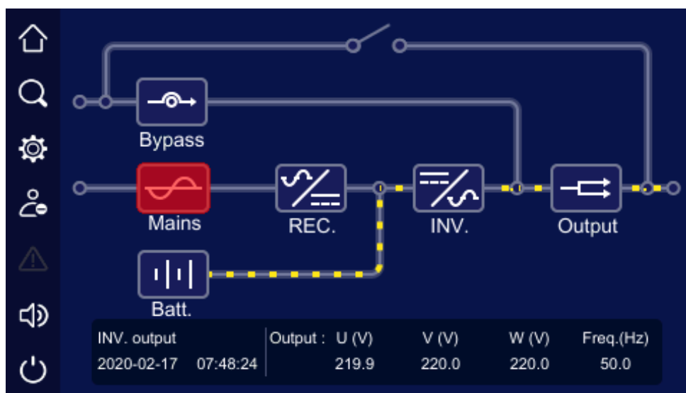
Рис 4.6 Сеть за пределами допусков, питание нагрузки от АКБ
