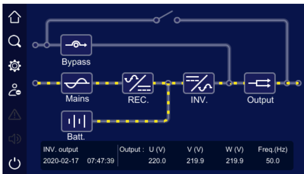
Рис 4.5 Сеть в норме, работа нагрузки от инвертора
