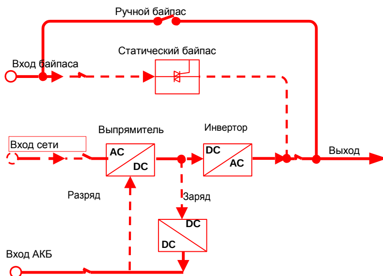
Рис 2-12 Режим ручного байпаса ((жирная линия показывает поток энергии))
