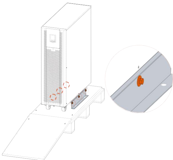
Рис. 3-5 Расположение болтов
