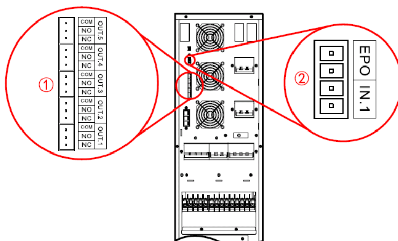
Рис 2-13 Расположение сухих контактов для ИБП 10/10S/15/15S/20/20S
