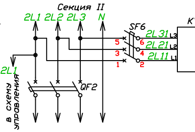
Схема подключения приводов силовых аппаратов приведена для моторных приводов Legrand DPX 1600 (26153)
