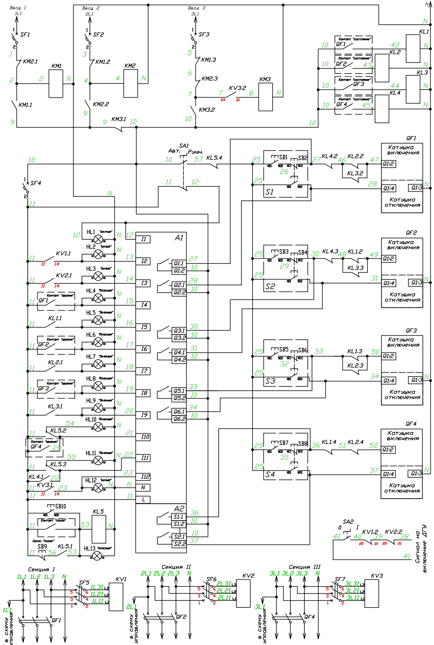
Схема подключения приводов силовых аппаратов приведена для моторных приводов Legrand DPX 1600 (26153)
