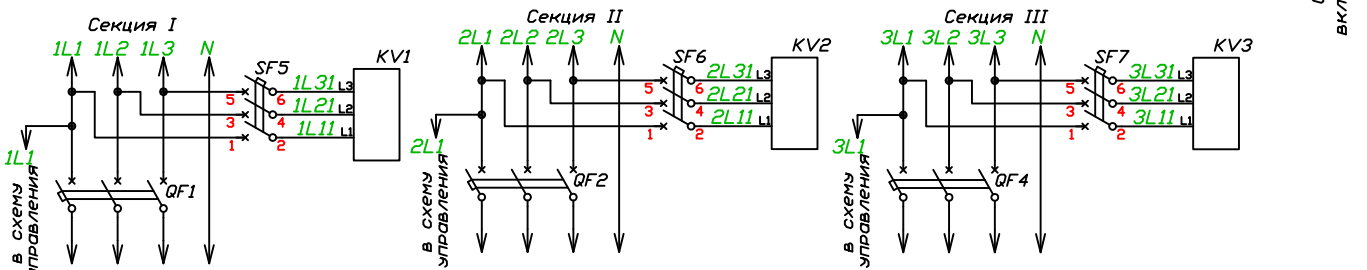
Схема подключения приводов силовых аппаратов приведена для моторных приводов EKF автоматов типа ВА-99М время паузы между отключением-включением привода 3с и для моторных приводов CHINT автоматов типов NM1-63, NM1-630, NM8(S)-125, NM8(S)-630, время паузы между отключением-включением привода 3с
