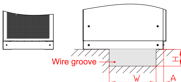
Рис3-15 Канал для прокладки кабелей
