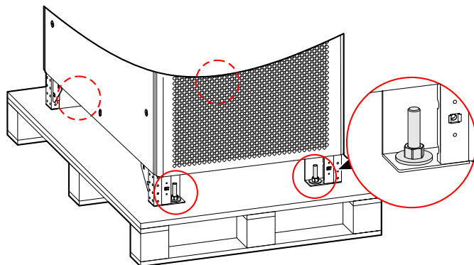
Рис3-8 Расположение крепёжных болтов МУ33160, МУ33200
