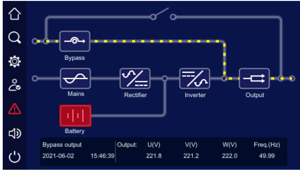
Рис4-5 Батарея неисправна, питание нагрузки через байпас
