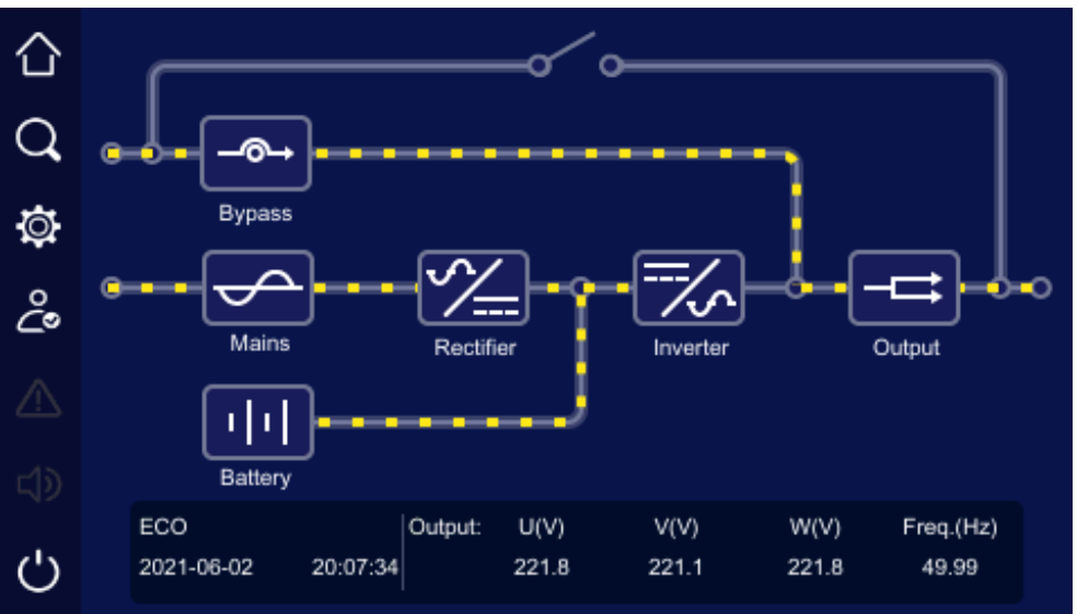
Рис4-9 ИБП работает в режиме ECO
