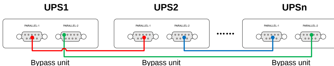
Рис2-13 Соединение портов RS485 нескольких параллельно работающих ИБП. (На рис показано соединение портов параллельной работы PARALLEL1 и PARALLEL2, порты RS485 соединяются точно так же)
