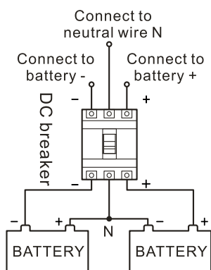
Рис3-38 Схема подключения аккумуляторной батареи
