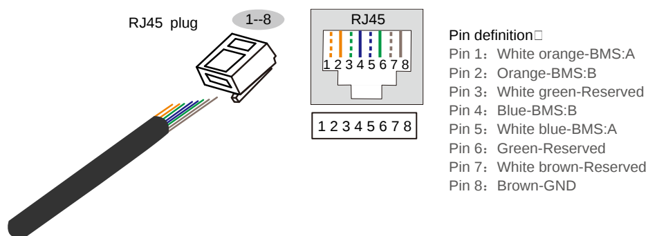
Рис2-20 Назначение контактов порта BMS
