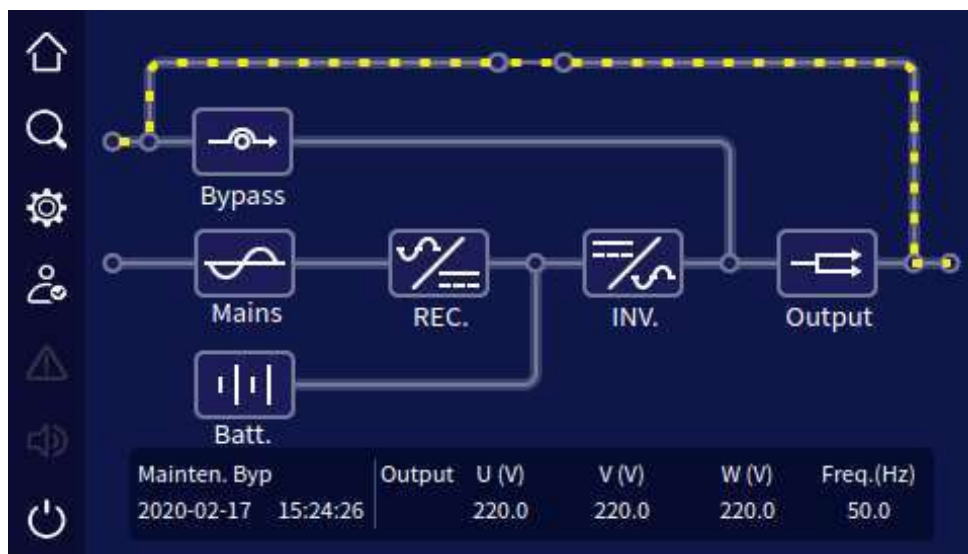
Рис4-11 ИБП работает через сервисный байпас
