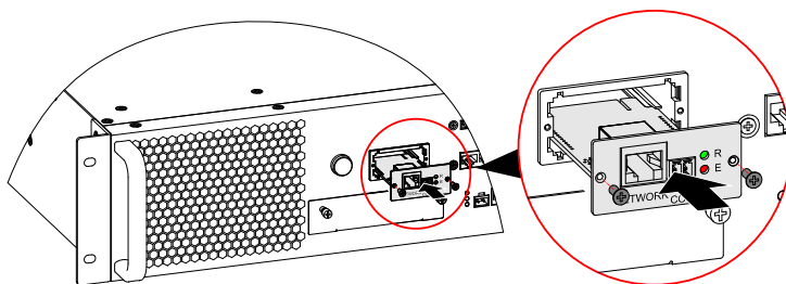
Рис3-22 Установка платы SNMP
