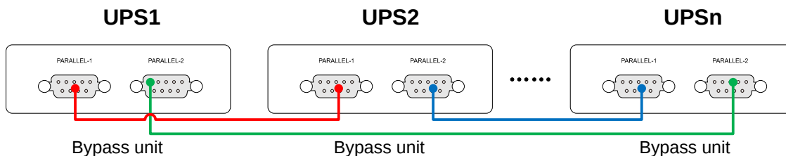
Рис2-21. Подключение кабелей параллельной работы. В системе несколько ИБП
