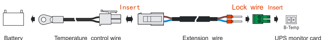
Рис2-23. Подключение датчика термокомпенсации
