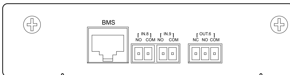
Рис2-19 Плата BMS
