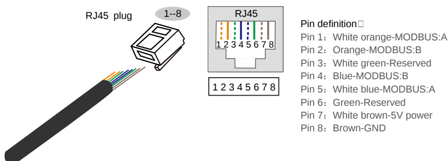
Рис2-14 Назначение контактов порта MODBUS
