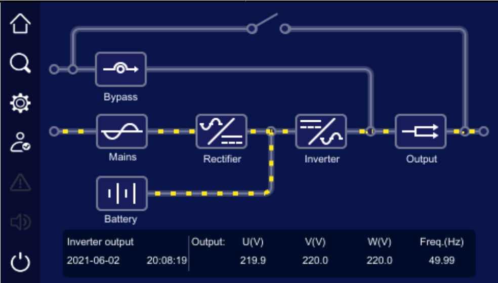
Рис4-7 ИБП работает в режиме двойного преобразования
