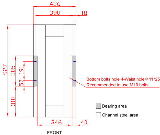
Рис3-11 Рекомендованные размеры стальных швеллеров, размеры в мм.
