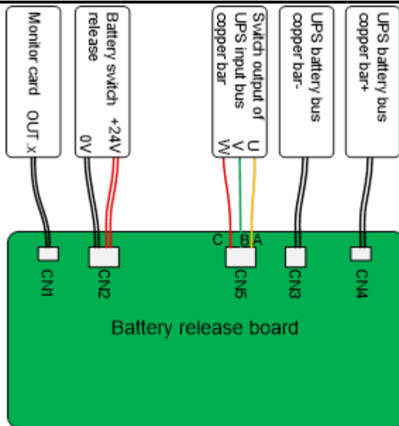
Рис3-27 Подключение платы устройства управления размыкателем цепи батареи
