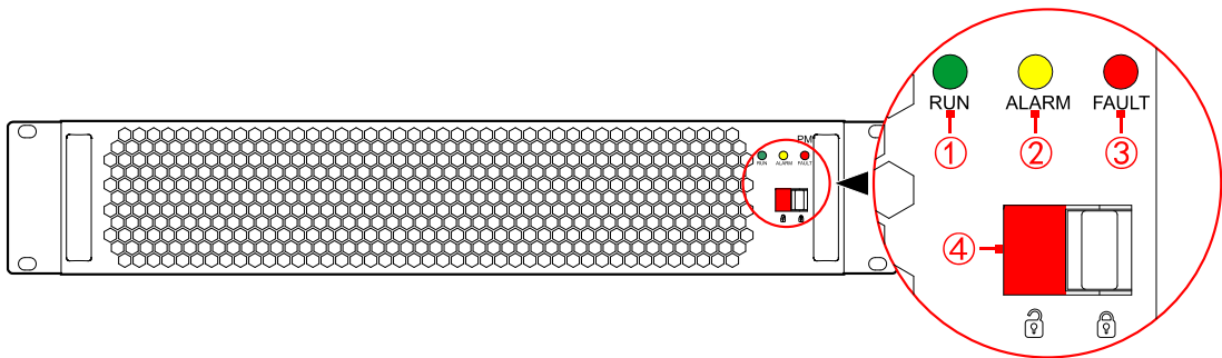
Рис2-9 Внешний вид силового модуля
