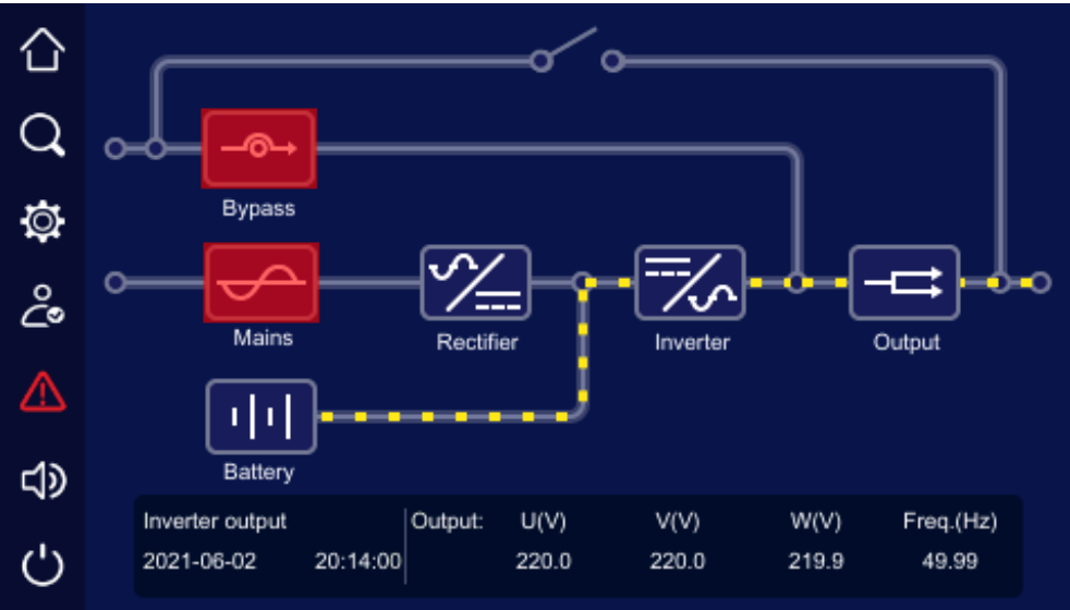
Рис4-6 Сеть и байпас за пределами допусков, инвертор питается от батареи
