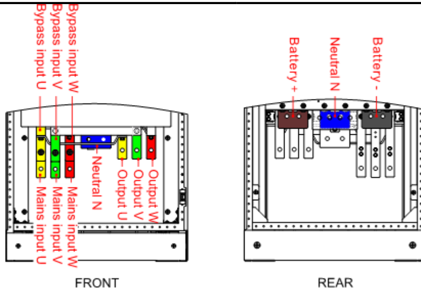
Рис3-36 Клеммы подключения МУ160, МУ200
