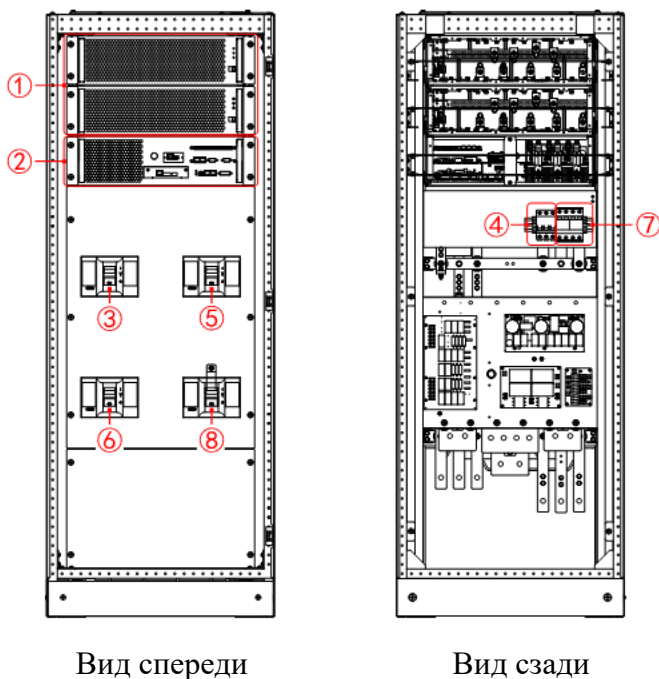
Рис2-8 Расположение основных элементов в ИБП МУ160-200 (дверца ИБП открыта)
