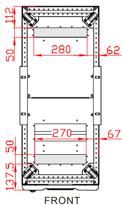
Рис3-29 Расположение кабельных проемов в нижней части ИБП МУ60, МУ80, МУ100, МУ120
