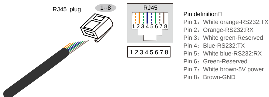
Рис2-15 Назначение контактов порта RS232
