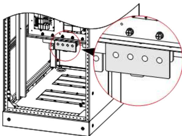
Рис3-35 Расположение шины РЕ ИБП МУ160, МУ200
