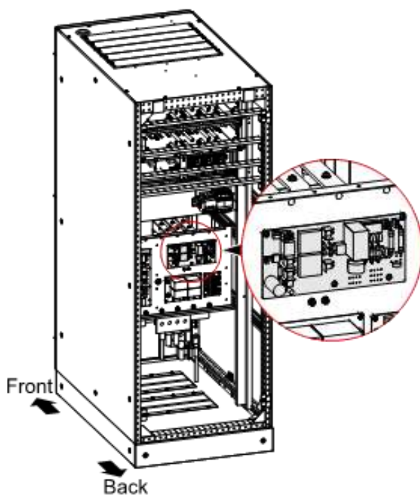
Рис3-26 Установка платы устройства управления размыкателем цепи батареи МУ160, МУ200
