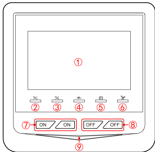
Рис2-5 Панель управления МУ60-120
