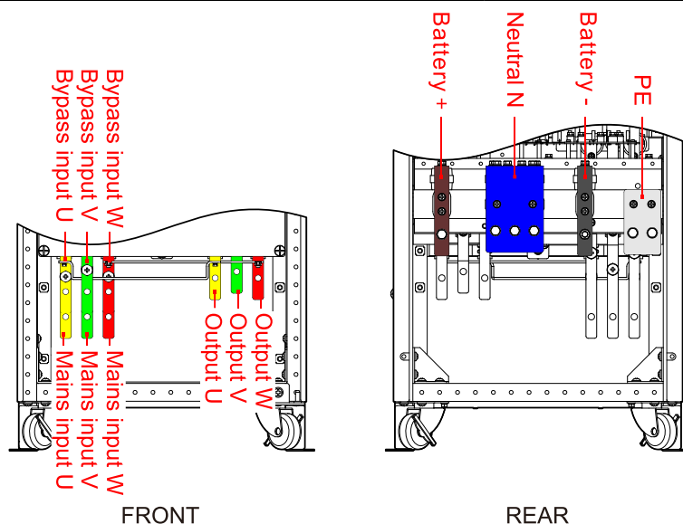
Рис3-30 Клеммы подключения MY60, MY80, MY100, MY120
