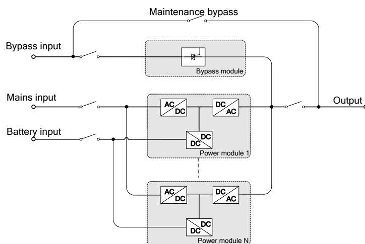
Рис2-2 Принципиальная схема работы ИБП
