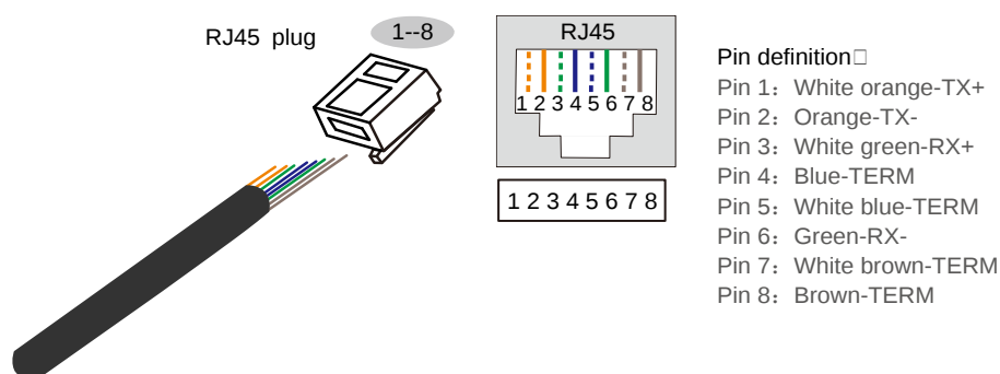
Рис2-17 Назначение контактов порта NETWORK
