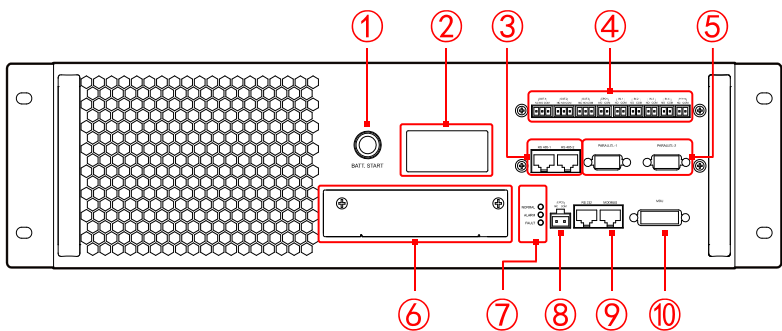
Рисунок2-7 Внешний вид модуля байпаса
