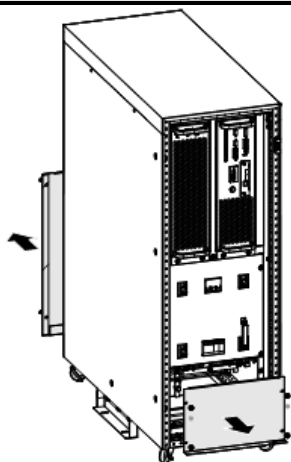
Рис3-28 Снятие панелей, закрывающих кабельные подключения
