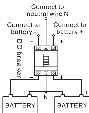
Рис3-32 Схема подключения аккумуляторной батареи
