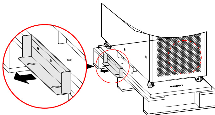
Рис3-7 Снятие монтажного кронштейна МУ3360, МУ3380, МУ33100, МУ120
