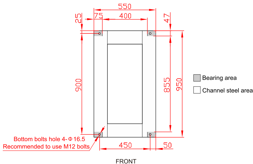
Рис3-18 Рекомендованные размеры стальных швеллеров, размеры в мм.
