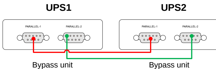
Рис2-21. Подключение кабелей параллельной работы. В системе два ИБП
