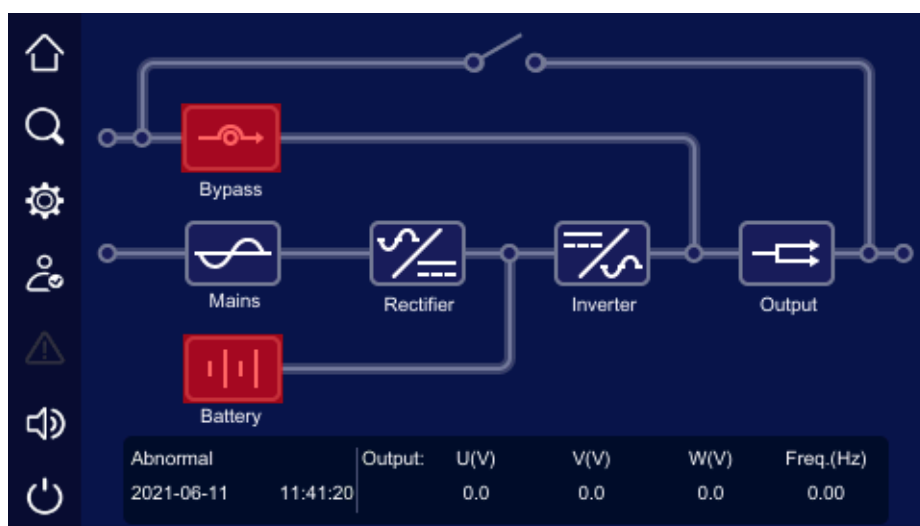
Рис4-3 Защита активна (без передачи энергии)
