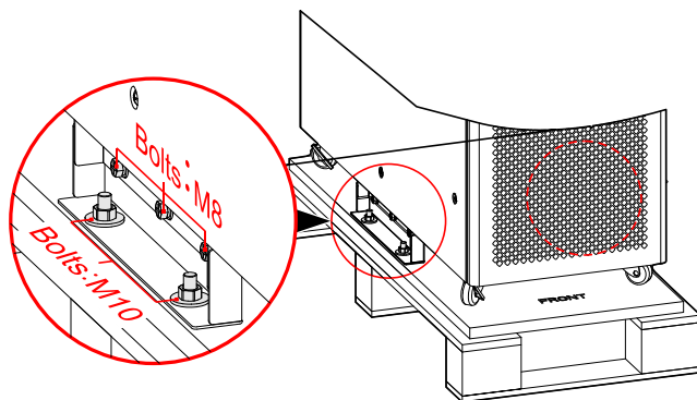
Рис3-6 Расположение крепёжных болтов МУ3360, МУ3380, МУ33100, МУ120
