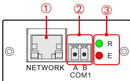
Рис 2-18 SNMP плата
