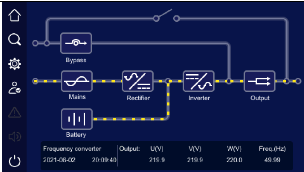
Рис4-10 ИБП работает в режиме конвертора частоты
