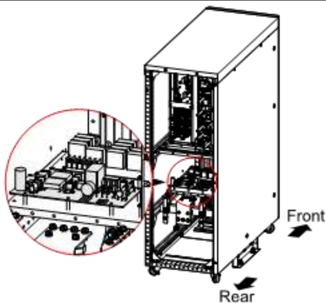
Рис3-25 Установка платы устройства управления размыкателем цепи батареи МУ60, МУ80, МУ100, МУ120
