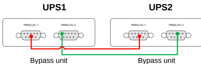
Рис2-12 Соединение портов RS485 двух параллельно работающих ИБП. (На рис показано соединение портов параллельной работы PARALLEL1 и PARALLEL2, порты RS485 соединяются точно так же)
