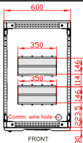
Рис3-34 Расположение кабельных проемов в нижней части ИБП МУ160, МУ200
