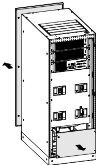
Рис3-33 Снятие панелей, закрывающих кабельные подключения МУ160, МУ200
