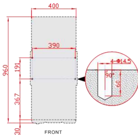
Рис3-10 Рама устройства и отверстия для монтажа в раме ИБП (вид снизу), размерность – мм.
