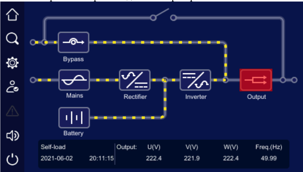
Рис4-8 ИБП работает в режиме самотестирования
