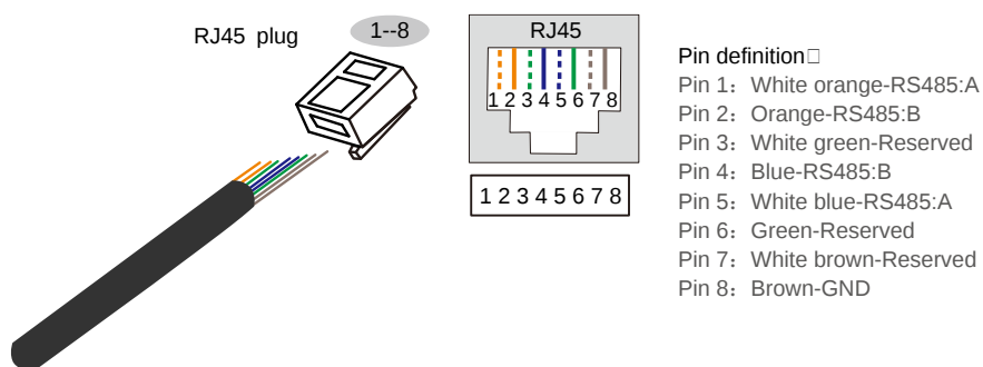
Рис2-11 Назначение контактов порта RS485
